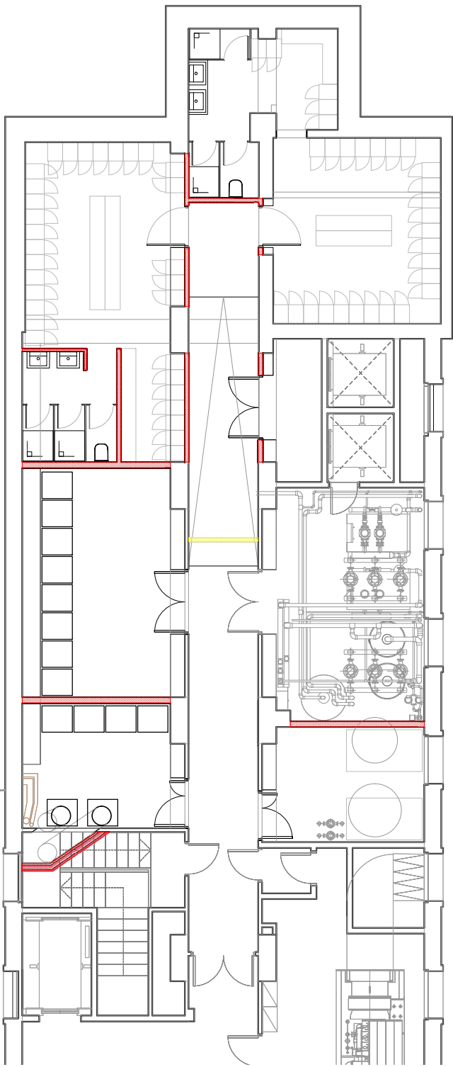
PS | PLANTA SOTERRANI - ENDERROC / OBRA NOVA REF-04 Esc: 1/100 (A3)
