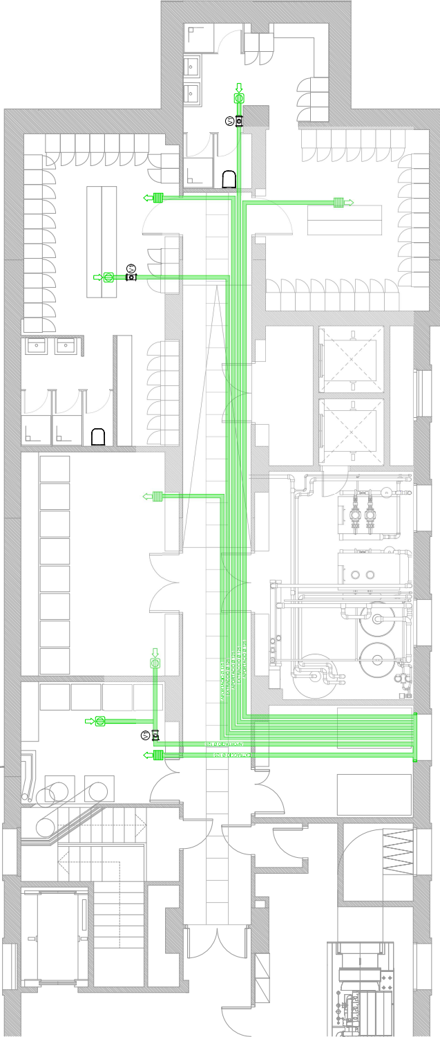
INS | PLANTA SOTERRANI - INSTAL·LACIÓ VENTILACIÓ INS-03 Esc: 1/100 (A3)
