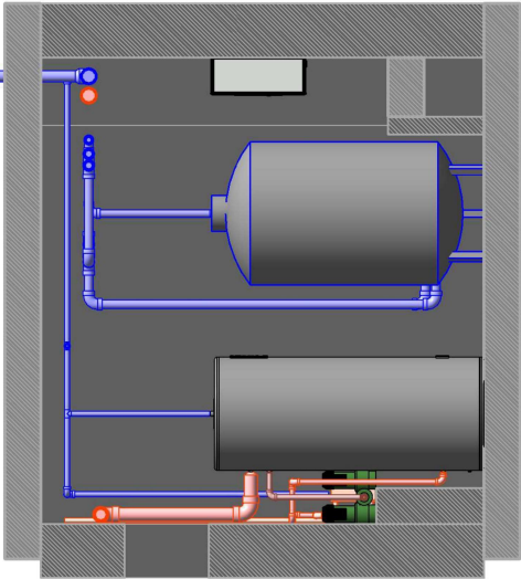
CAL | SALA DE TRACTAMENT AIGÜES - ALÇAT 2 INS-04 Esc: 1/50 (A3)
