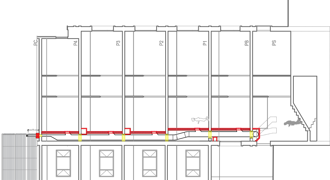
SEC-1 | SECCIÓ ÀMBIT ACTUACIÓ - ENDERROC / OBRA NOVA REF-44 Esc: 1/150 (A3)
