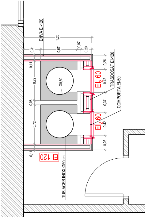
PT REF-03 PLANTA TIPO CONDUCTO Esc: 1/30 (A3)
