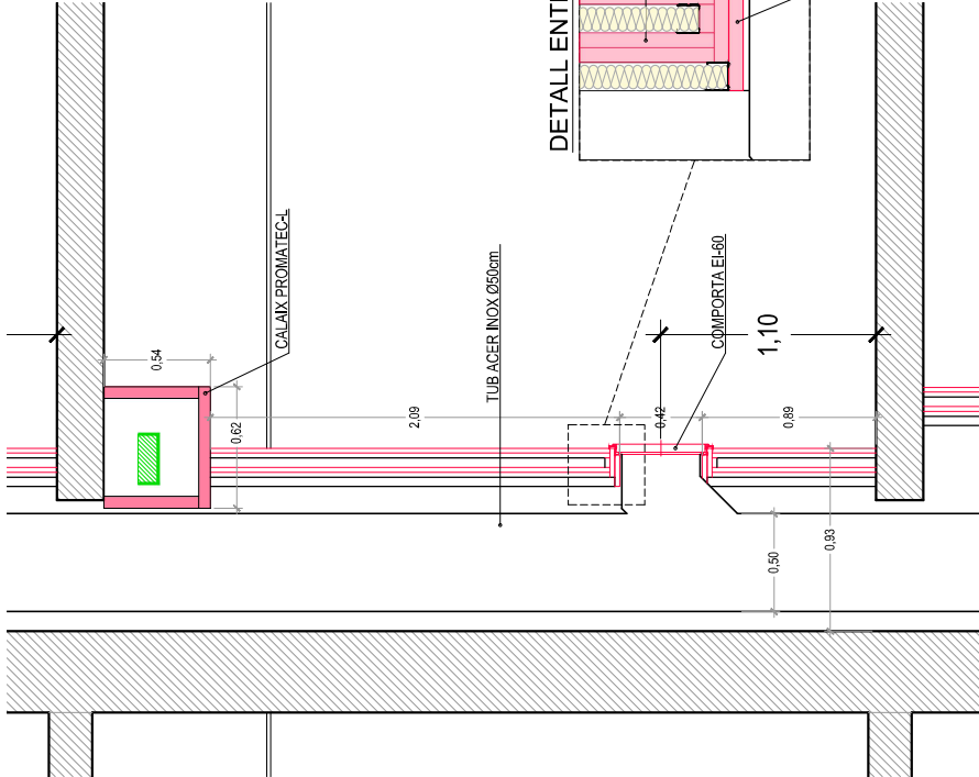
S1 REF-03 SECCIÓ CONDUCTE Esc: 1/30 (A3)
