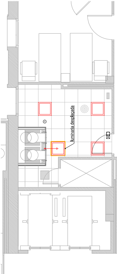
P8 | P8-INSTAL·LACIÓ ELÈCTRICA INS-02 Esc: 1/75 (A3)
