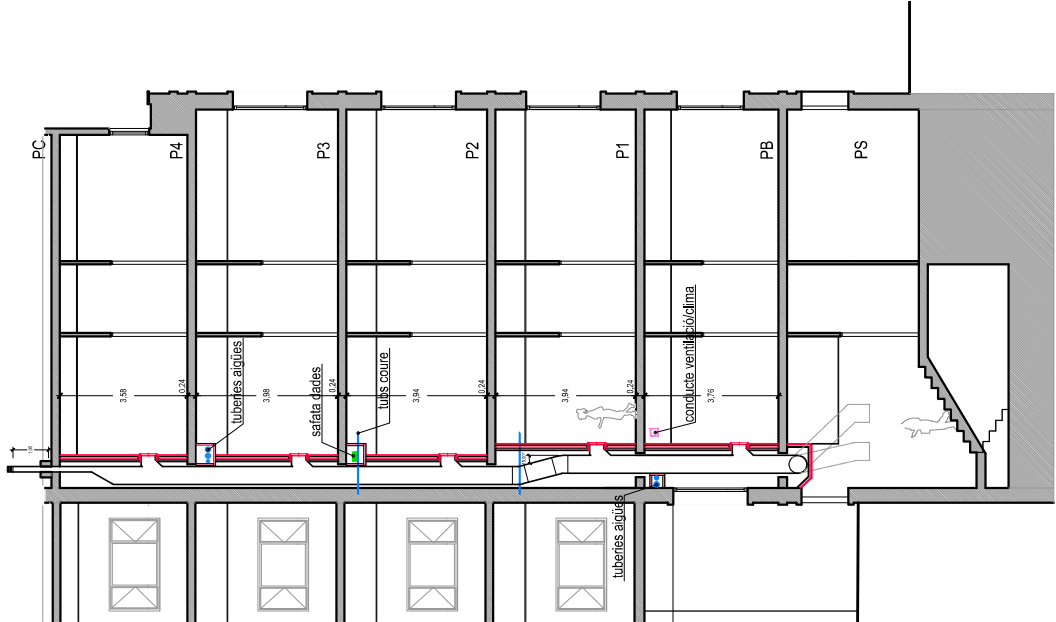
SEC-1 | SECCIÓ AMBIT ACTUACIÓ - ESTAT REFORMAT REF-01 Esc: 1/150 (A3)
