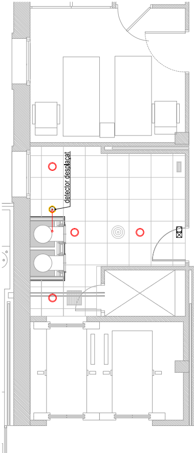
P1 | P1-INSTAL·LACIÓ ELÈCTRICA INS-02 Esc: 1/75 (A3)
