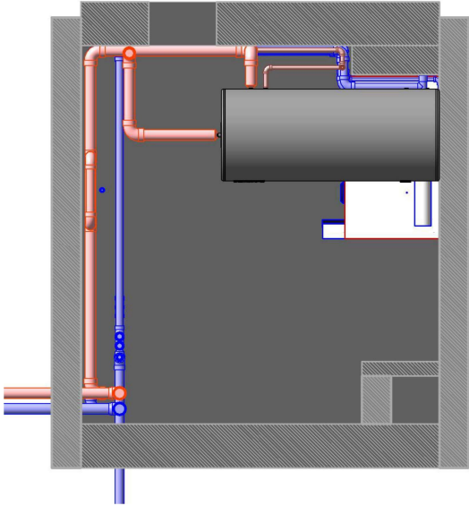
CAL | SALA DE TRACTAMENT AIGÜES - ALÇAT 5 INS-04 Esc: 1/50 (A3)
