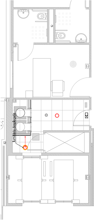
P3 | P3-INSTAL·LACIÓ ELÈCTRICA INS-02 Esc: 1/75 (A3)
