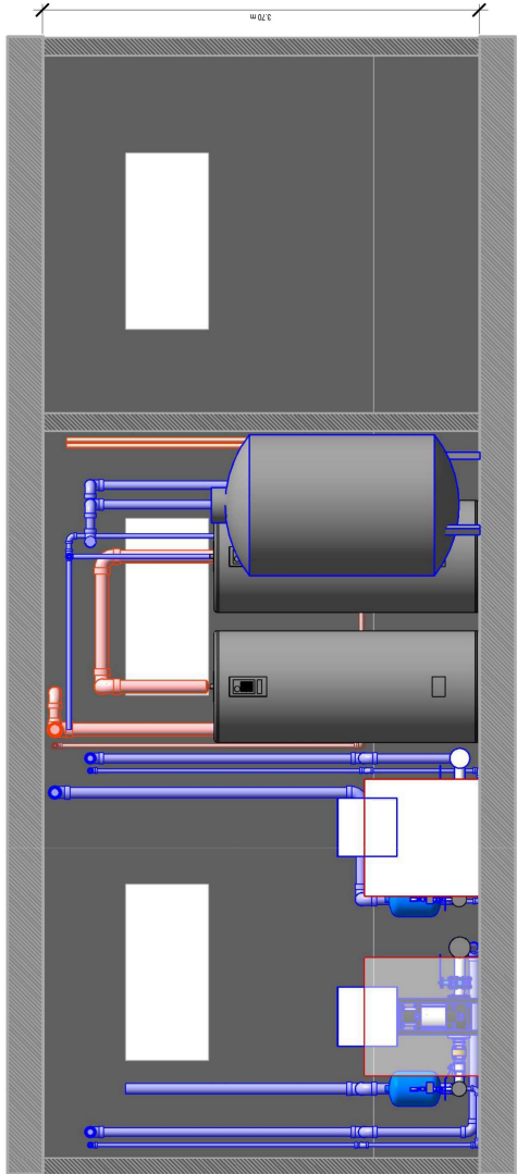
CAL | SALA DE TRACTAMENT AIGÜES - ALÇAT 5 INS-04 Esc: 1/50 (A3)
