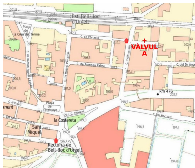
Imatge 1. Ubicació dels hidrants
