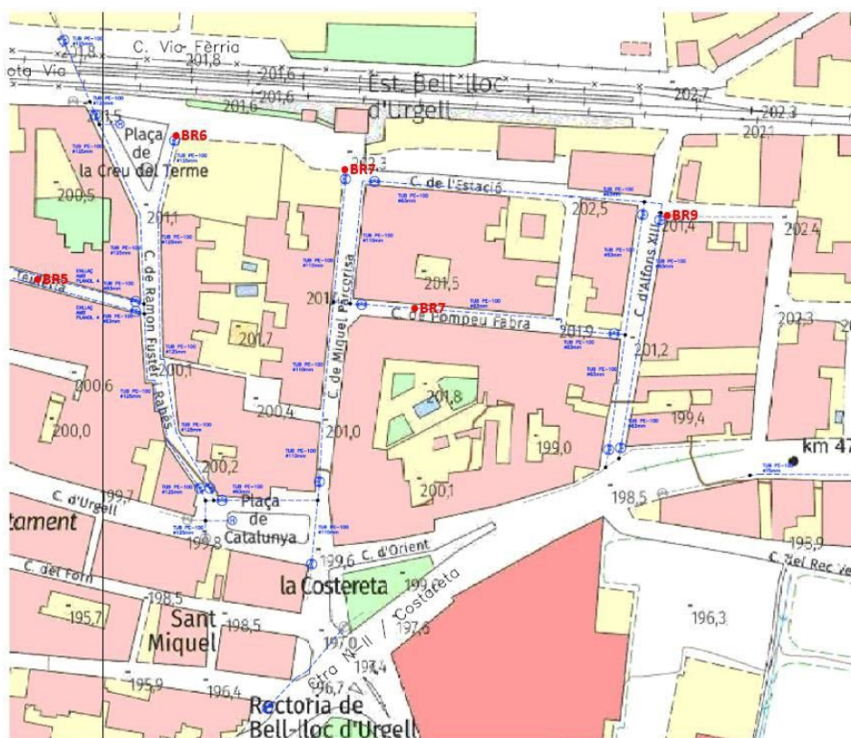
Imatge 4. Ubicació de les boques de reg 5-9
