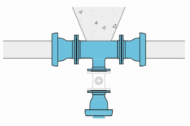
DETALL DE CONNEXIÓ A XARXA EXISTENT
