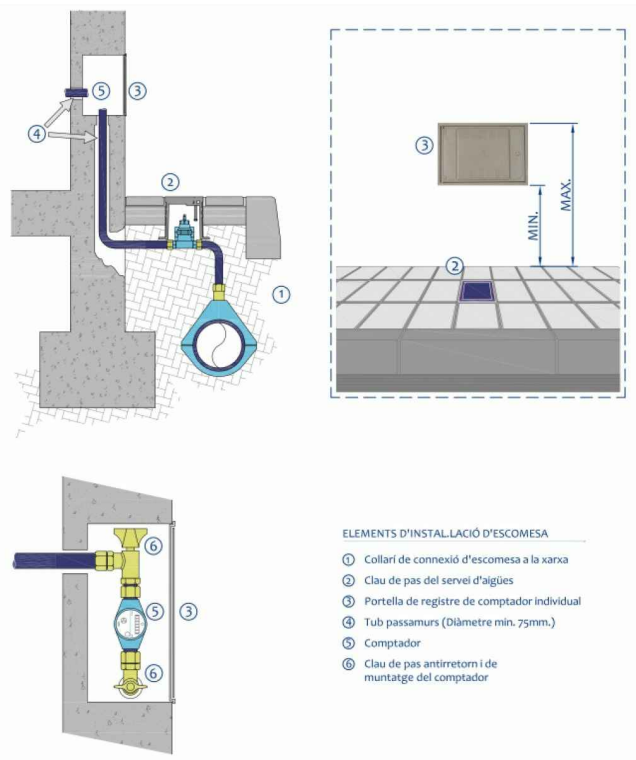
DETALL ESCOMESA
