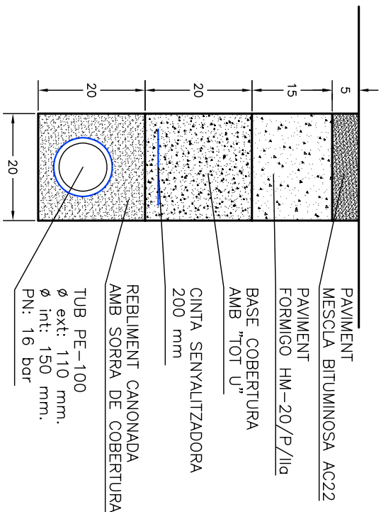
DETALL RASA PER CANONADA
