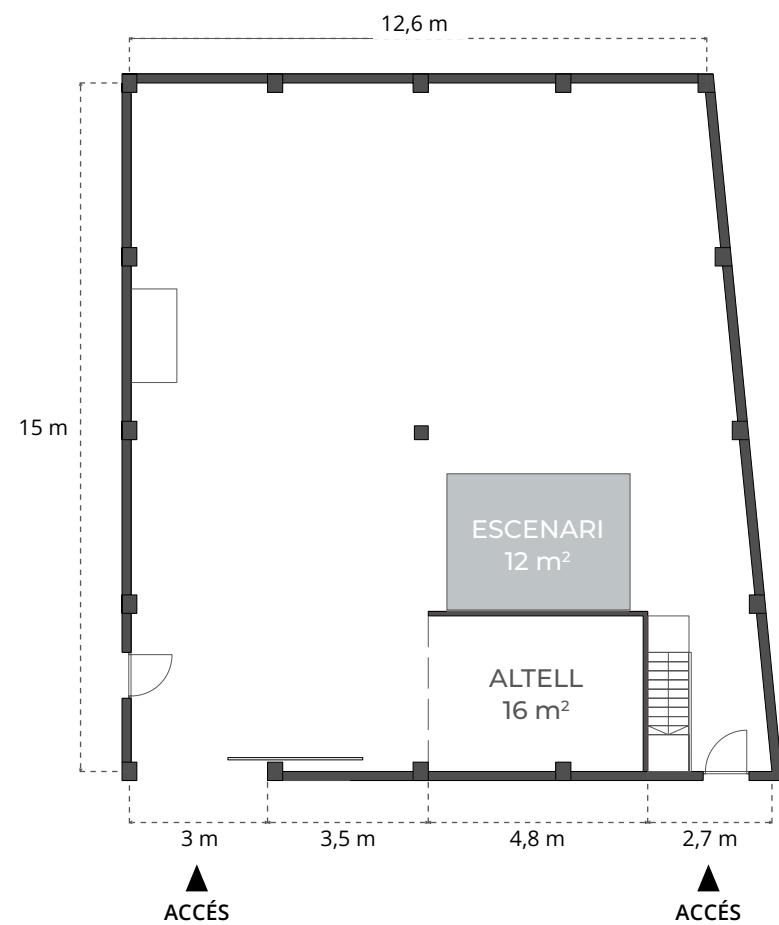
NAU BETOR / PLANTA BAIXA. ACCÉS PEL PASSATGE INTERIOR DE LA NAU BOSTIK.
