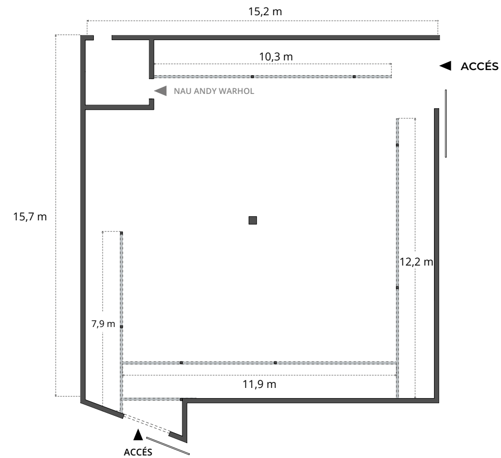
NAU PILAR VERS / PLANTA BAIXA. CONNECTADA AMB LA NAU ANDY WARHOL. ACCÉS PER CARRER PRINCIPAL DE NAU BOSTIK I PEL PASSATGE TRANSVERSAL.
