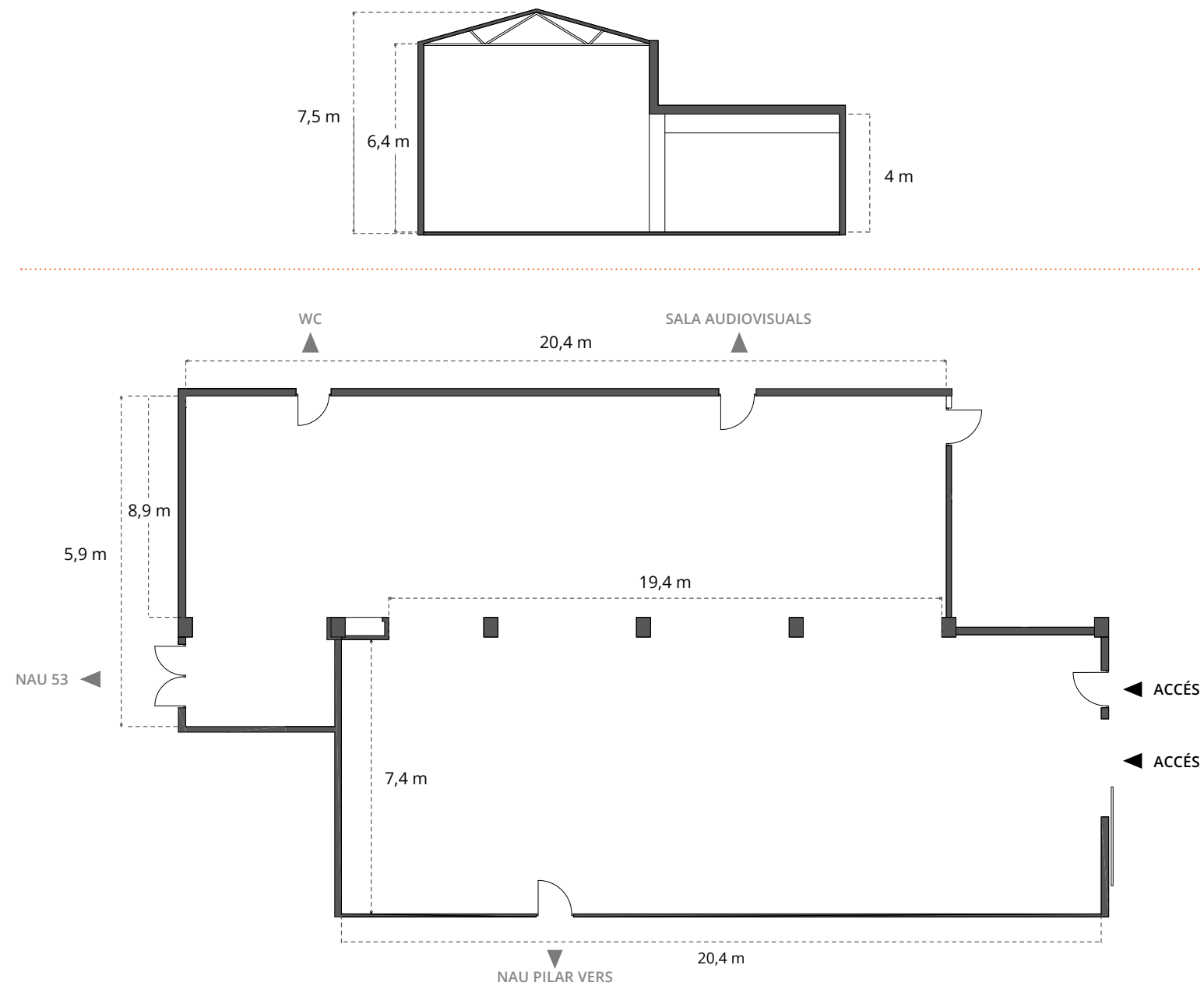
NAU ANDY WARHOL / PLANTA BAIXA. ACCÉS PEL CARRER PRINCIPAL DE LA NAU BOSTIK. CONNECTADA AMB LA NAU KM14 I LA SALA AUDIOVISUAL.
