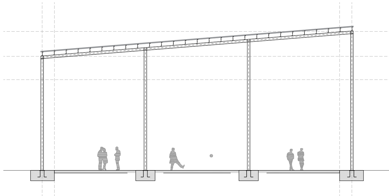
ALÇAT C-C'
