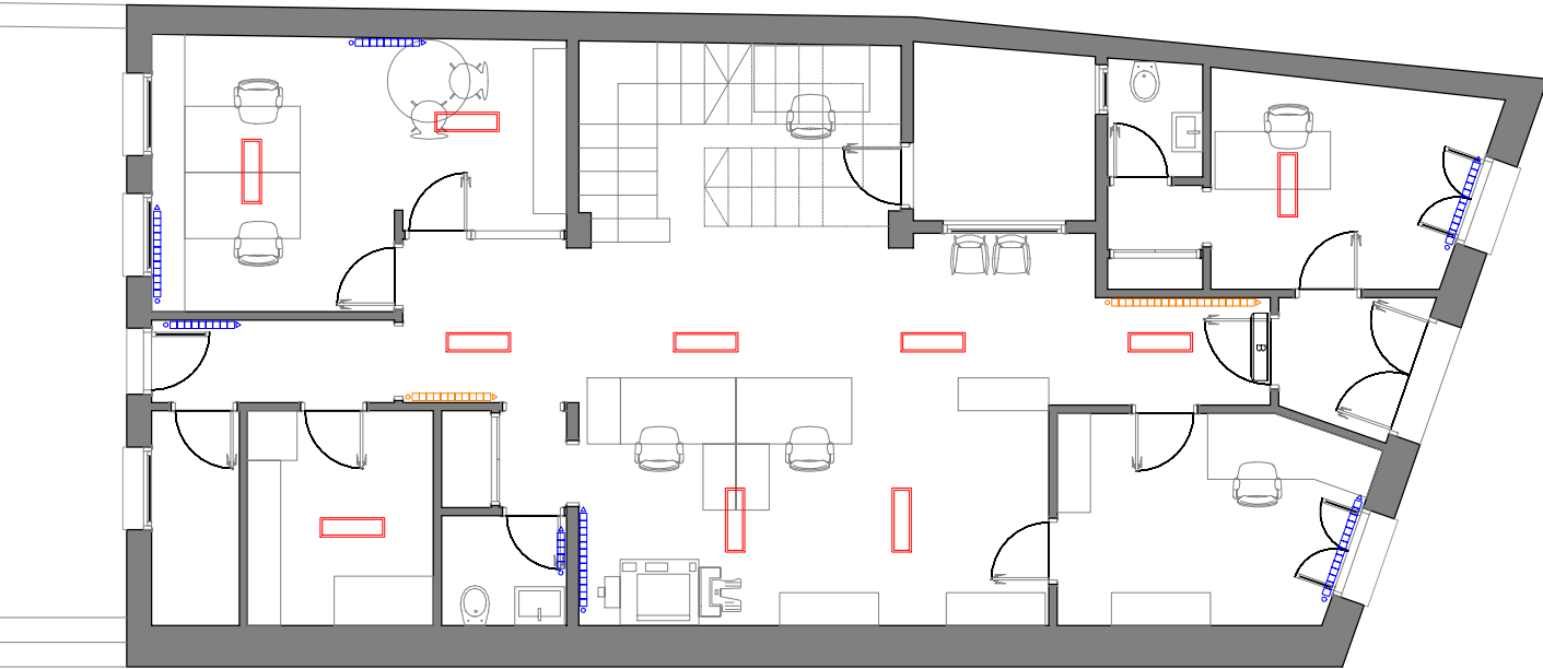
planta existent
