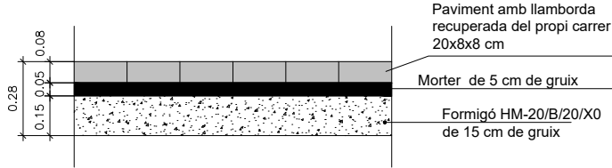
PAVIMENT AMB APLACAT DE PEDRA recuperada del propi carrer E:1/25
