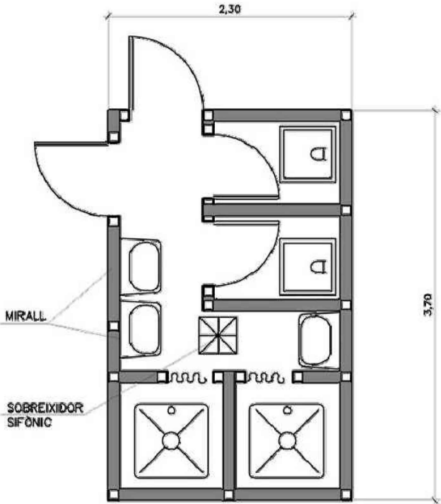
SERVEIS
