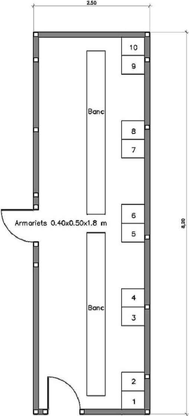
VESTIDORS
