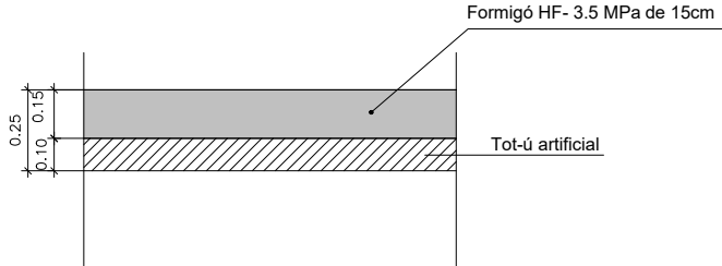
PAVIMENT DE FORMIGÓ HF-3.5 MPa E:1/25
