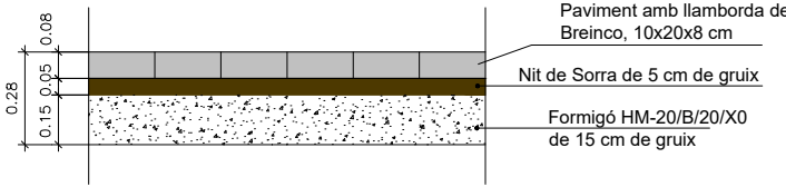
PAVIMENT AMB LLAMBORDA MODEL TARGA E:1/25
