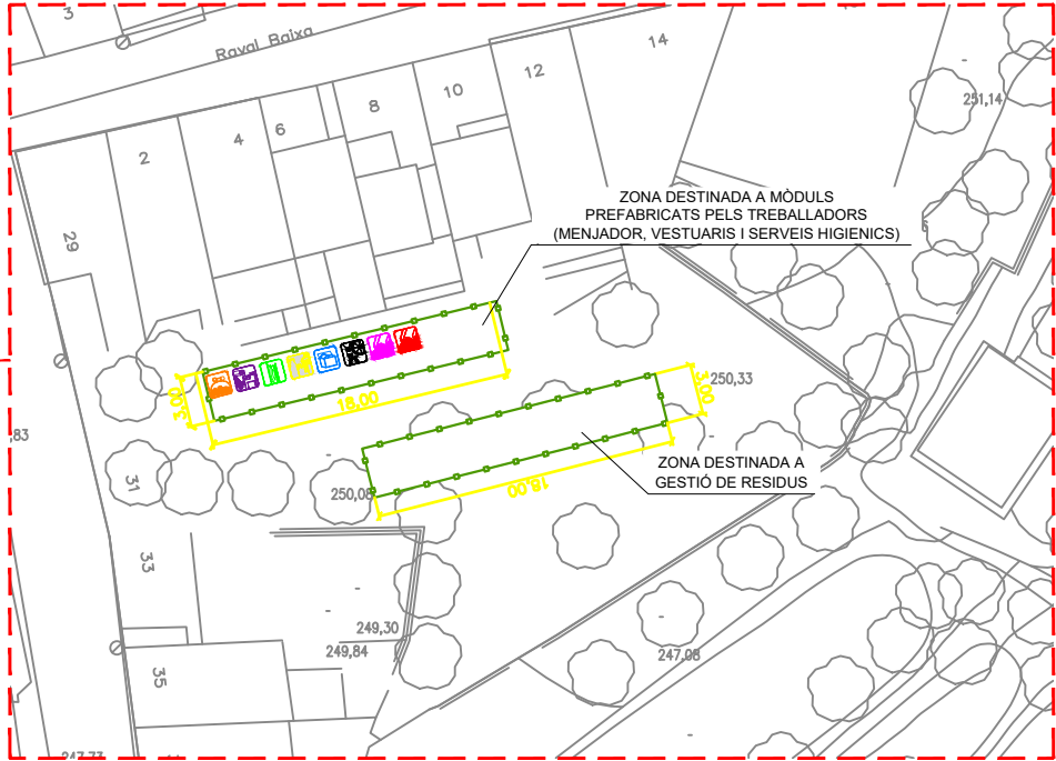
SITUACIÓ DE CASETES D'OBRA E:1/500
