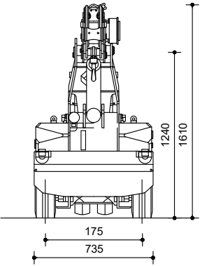
Mini grúa pack & carry elèctrica de 2.5T
