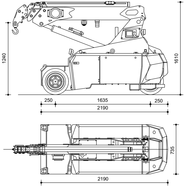
Maquinària de transport i càrrega E 1:40
