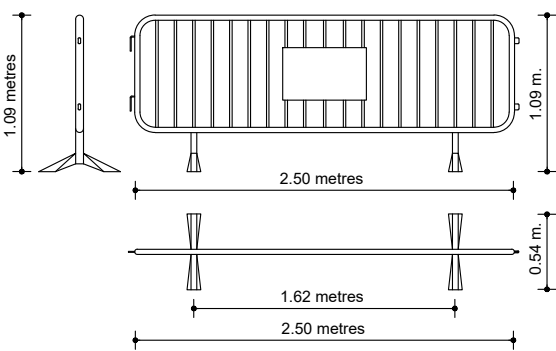
Tanca mòbil E 1:50
