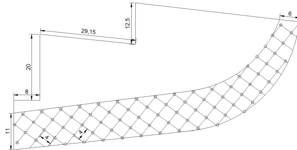
Imatge 6: Malla de cable d'acer de 12 mm en mòduls de 4 metres a l'àrea a intervenir.
