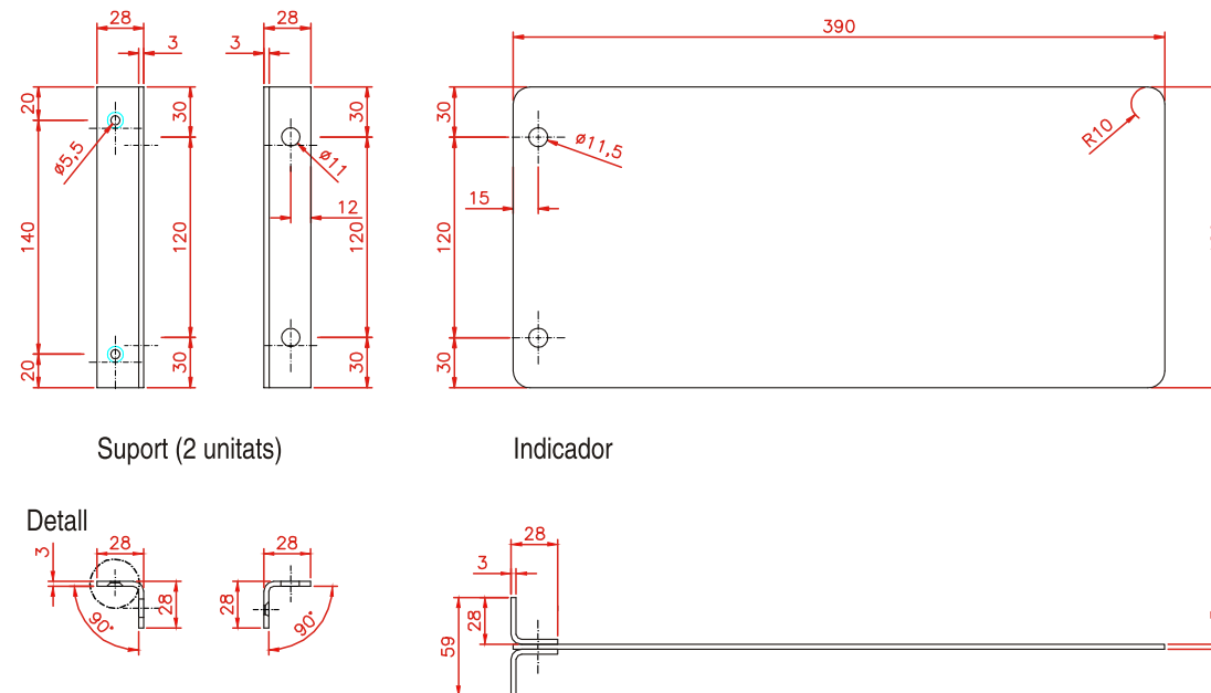
Detall forat passant
