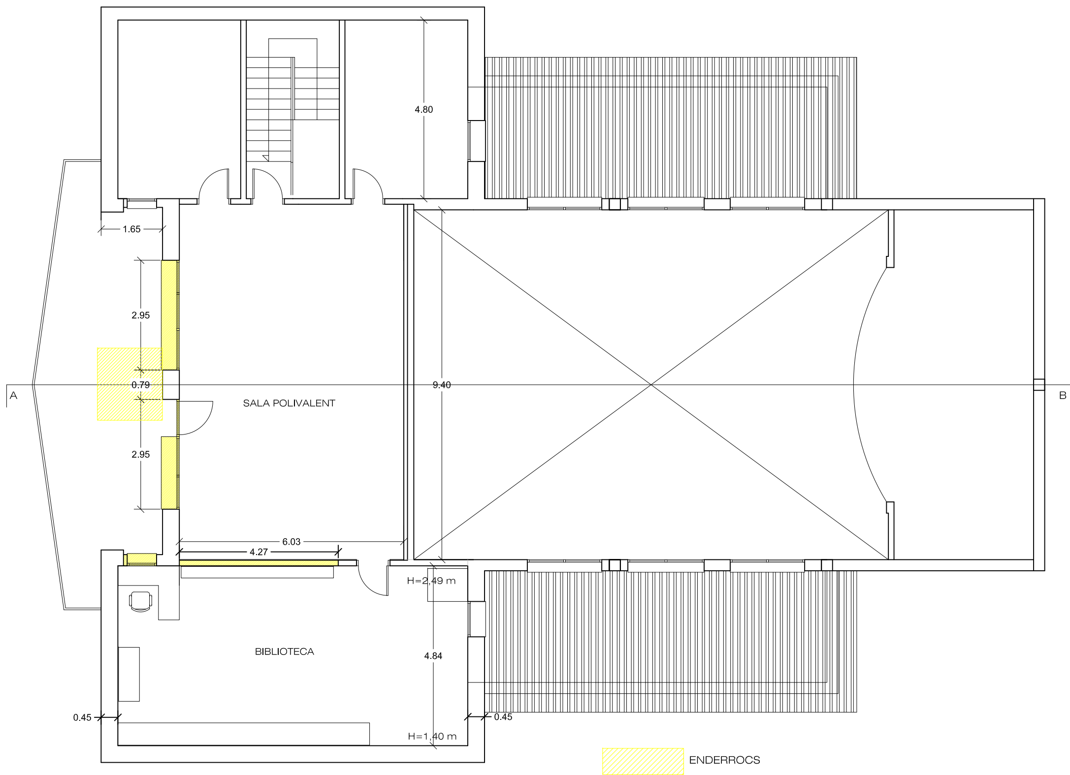
PLANTA PRIMERA
