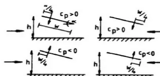
Fig. 10.3.2 - Hipòtesis de carga en marquesinas a una agua
