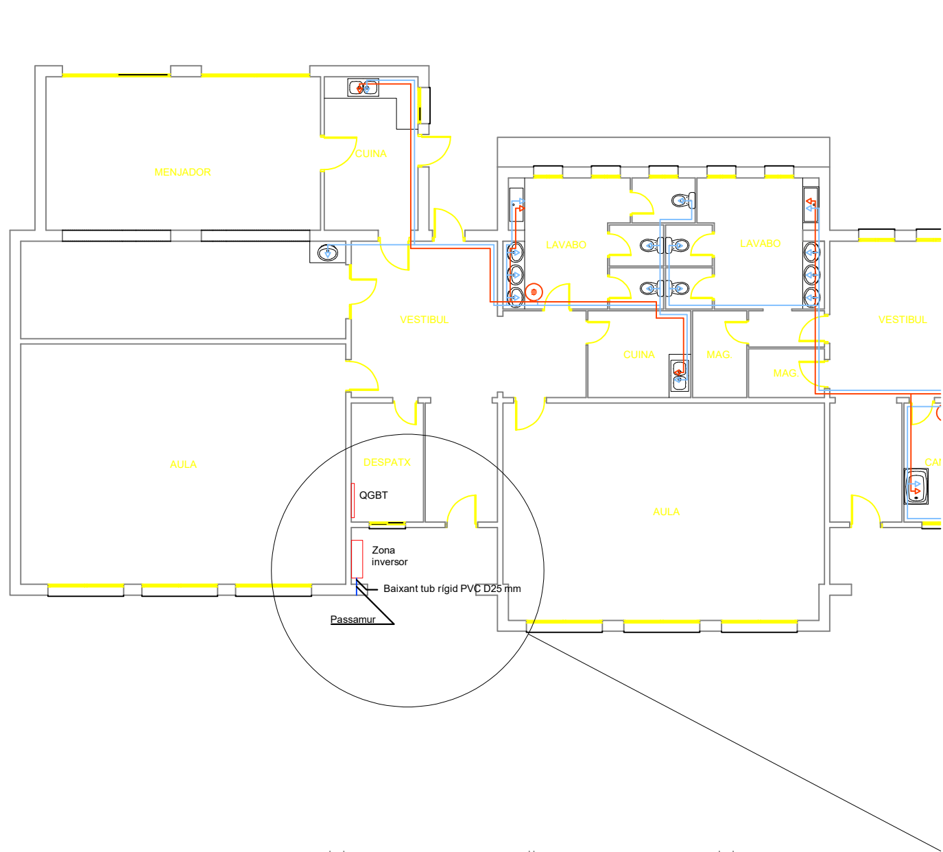
ESQUEMA PAS DEL CABLEJAT DE CORRENT CONTÍNUA INTERIOR
