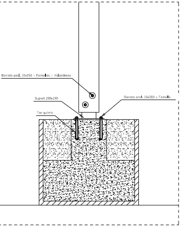
DETALL A , SUPORT PEUS DE PILAR
