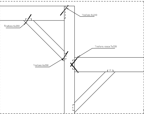
DETALL B , UNIONS CUES, TORNAPUNTES I JASSERES
