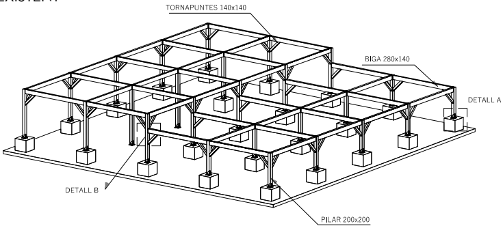
3D PÈRGOLA EXISTENT
