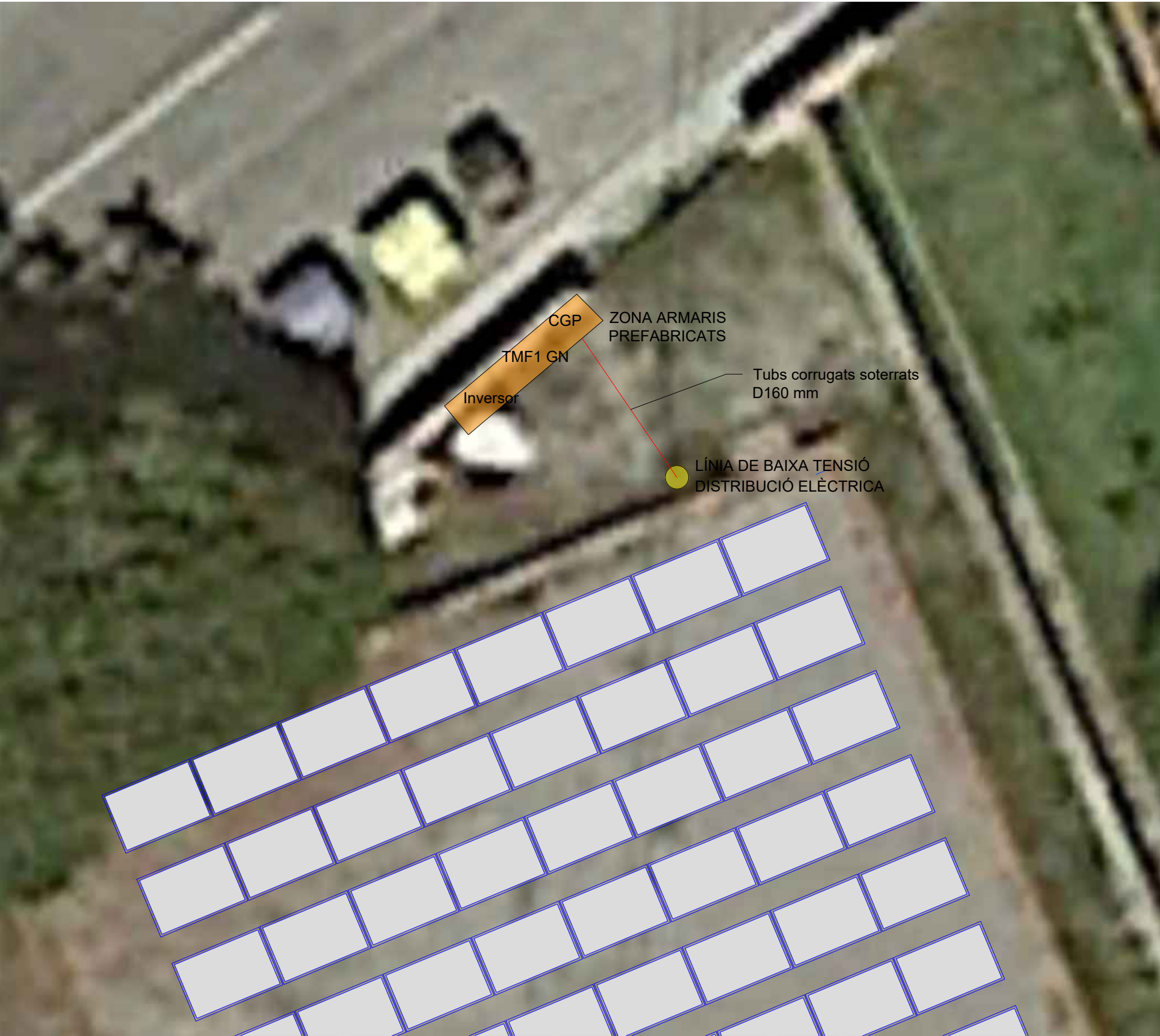
QUADRE SERVEIS GENERALS - ARMARIS PREFABRICATS
