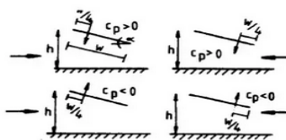
Fig. 10.3.2 – Hipòtesis de carga en marquesinas a una aigua
