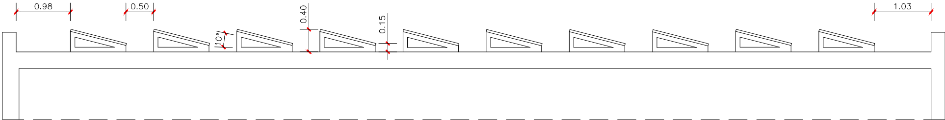
SECCIÓ A - A' COBERTA A
