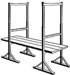
Fig. 1 b: Andamio de borriquetas verticales
