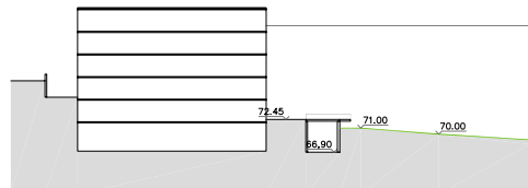
SECCIÒ J-J'
