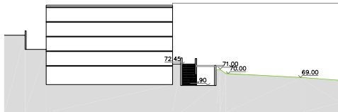
SECCIÒ I-I'
