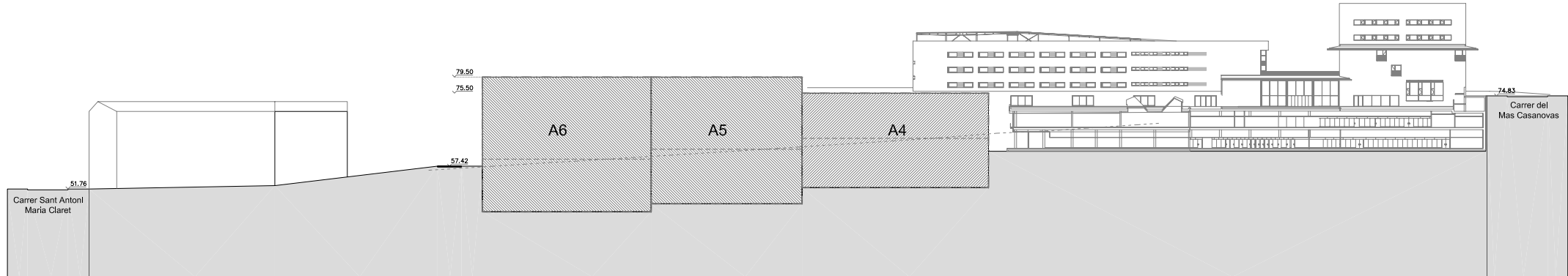
SECCIÒ E-E'
