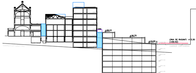
SECCIÒ H-H'
