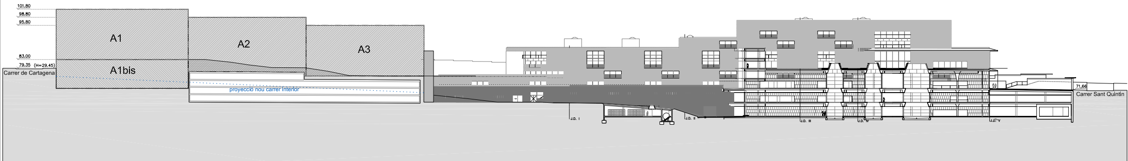
SECCIÒ B-B'
