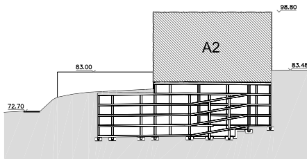
SECCIÒ F-F'
