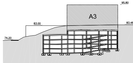
SECCIÒ G-G'
