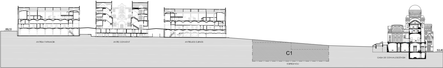
SECCIÒ D-D'
