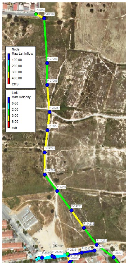
Figura 26. Resultats al tram 1 amb millores. Es representa cabal d'entrada als pous (l/s) i la velocitat del col·lector (m/s).
