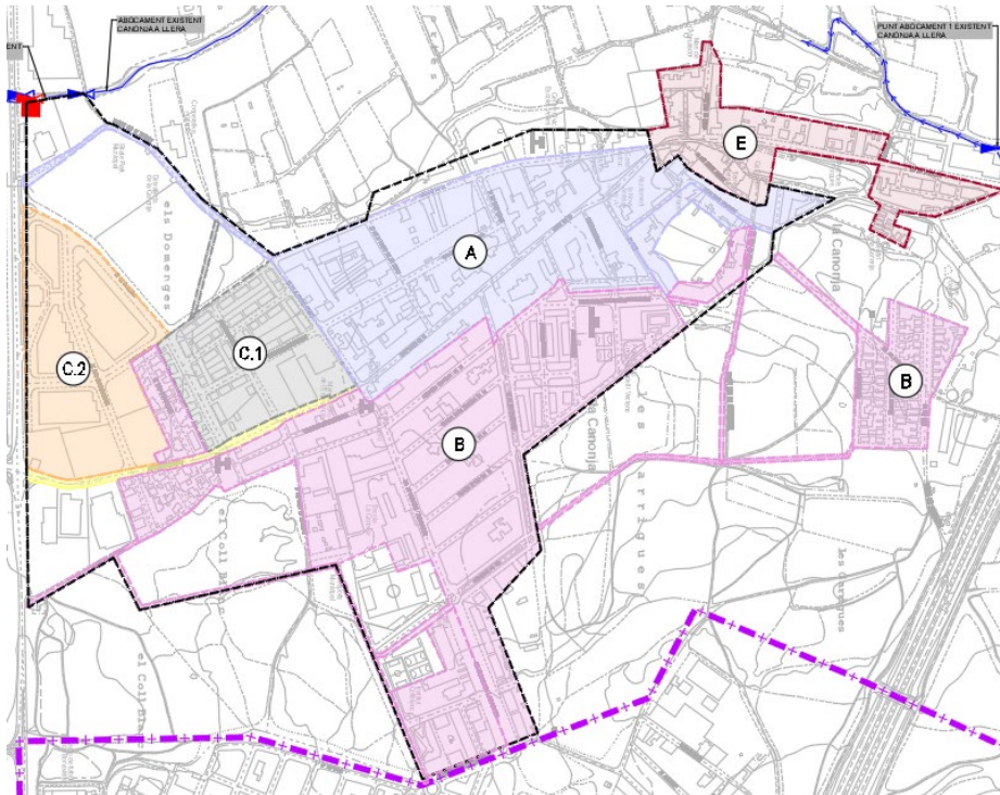
Figura 8. Discretització de les conques de l'àrea abastada per la xarxa de sanejament de La Canonja.
