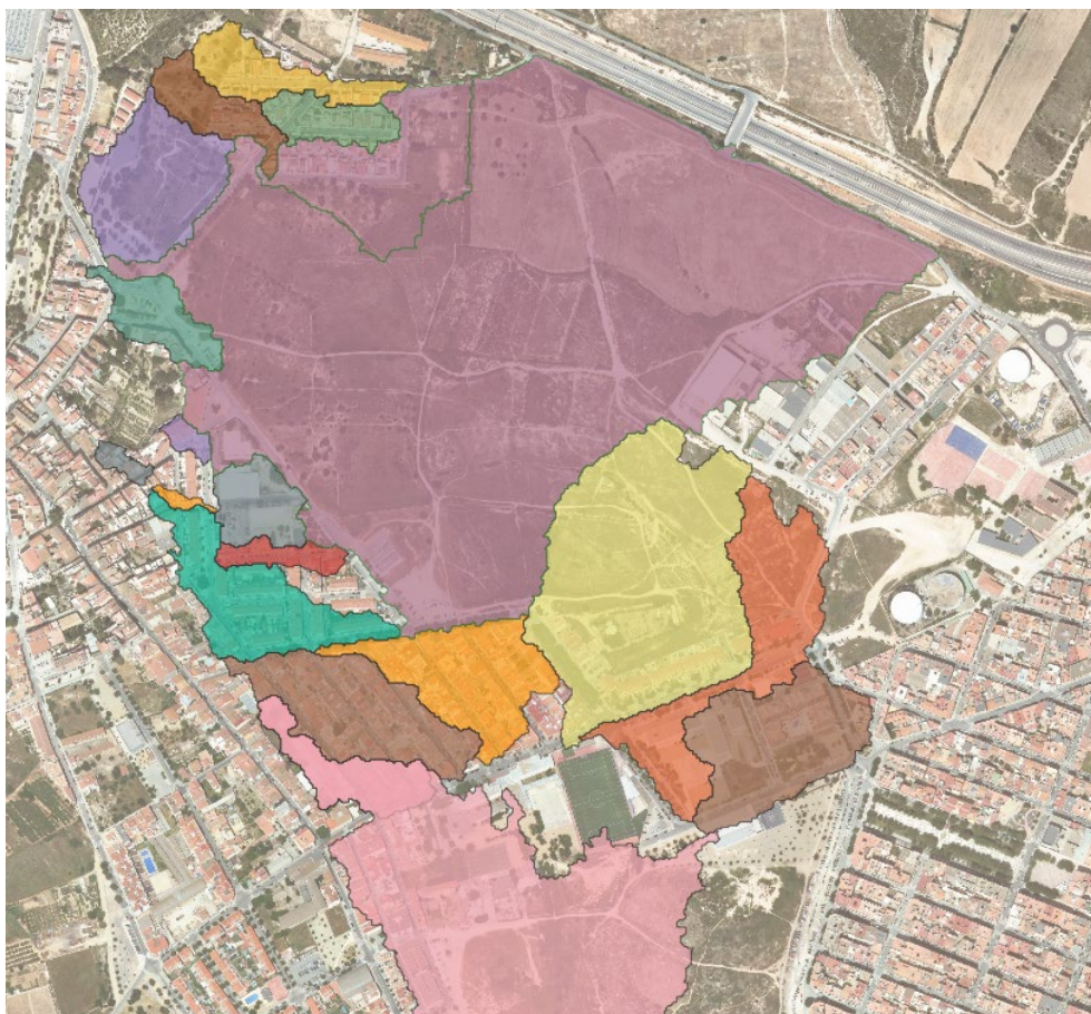
Figura 10. Obtenció de conques d'aigües pluvials per mitjà de software GIS.
