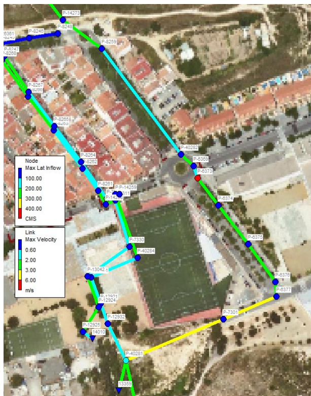
Figura 36. Resultats al tram 2 i 3 amb millores. Es representa cabal d'entrada als pous (l/s) i la velocitat del col·lector (m/s).
