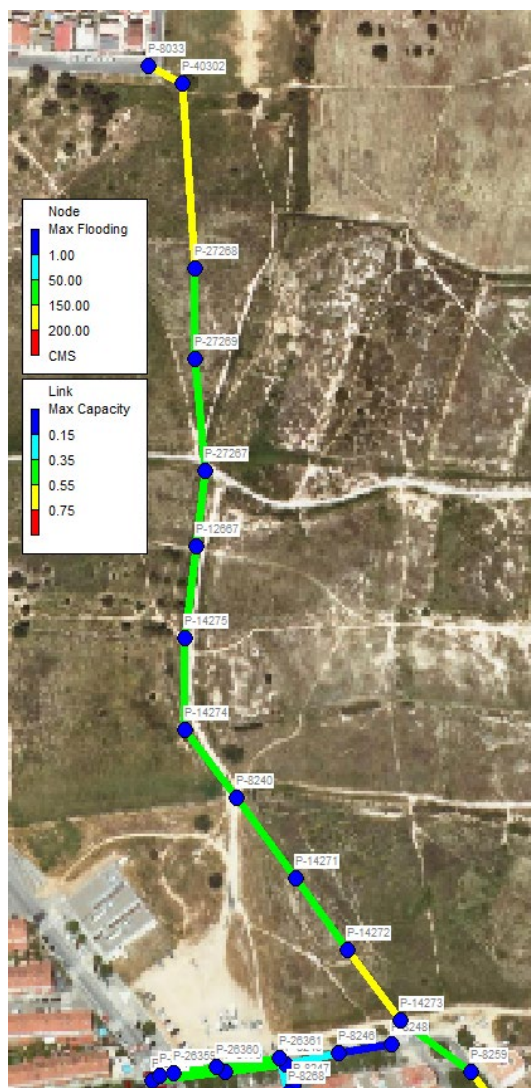
Figura 25. Resultats al tram 1 amb millores. Es representa el cabal sobreexidor dels pous (l/s) i la ocupació del col·lector (tant per u).
