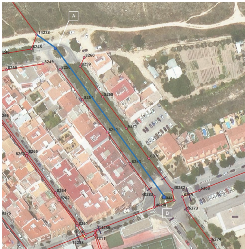
Figura 22. Alternativa a) de connexió del pou 6542 i col·lector del tram sud de l'av. de Collblanc.
