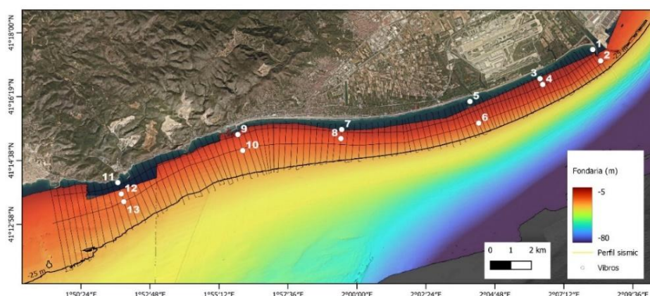
Figura 1. Localització dels 13 Vibrocores a realitzar entre el port de Barcelona i el port d'Aiguadolç.
