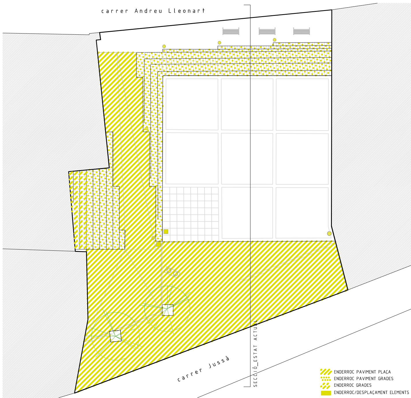
ESTAT ACTUAL_ENDERROC
