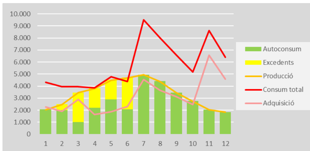
KIT AUTOCONSUM DE 20KW (Potència instal·lada 29,44kWp)
