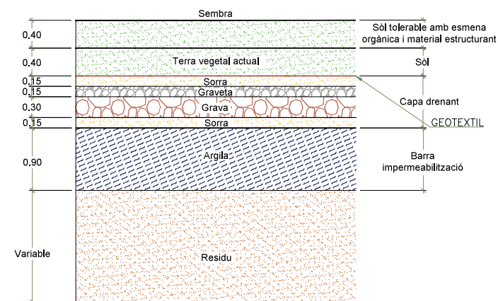
SECCIÓ TIPUS ESTÀNDAR DEL SEGELLAT ESCALA 1/50
