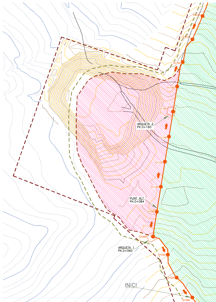
RESSEGELLAT, DEFINICIÓ ZONA VIALS. PLANTA ESCALA 1/1000
