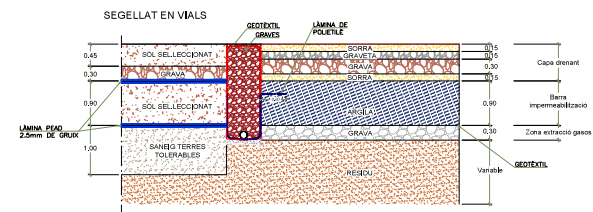
TRANSICIÓ ENTRE EL SEGELLAT STANDARD I EL DE VIALS. ESCALA 1/100
