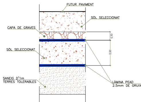
SEGELLAT EN ZONA DE VIALS. ESCALA 1/50
