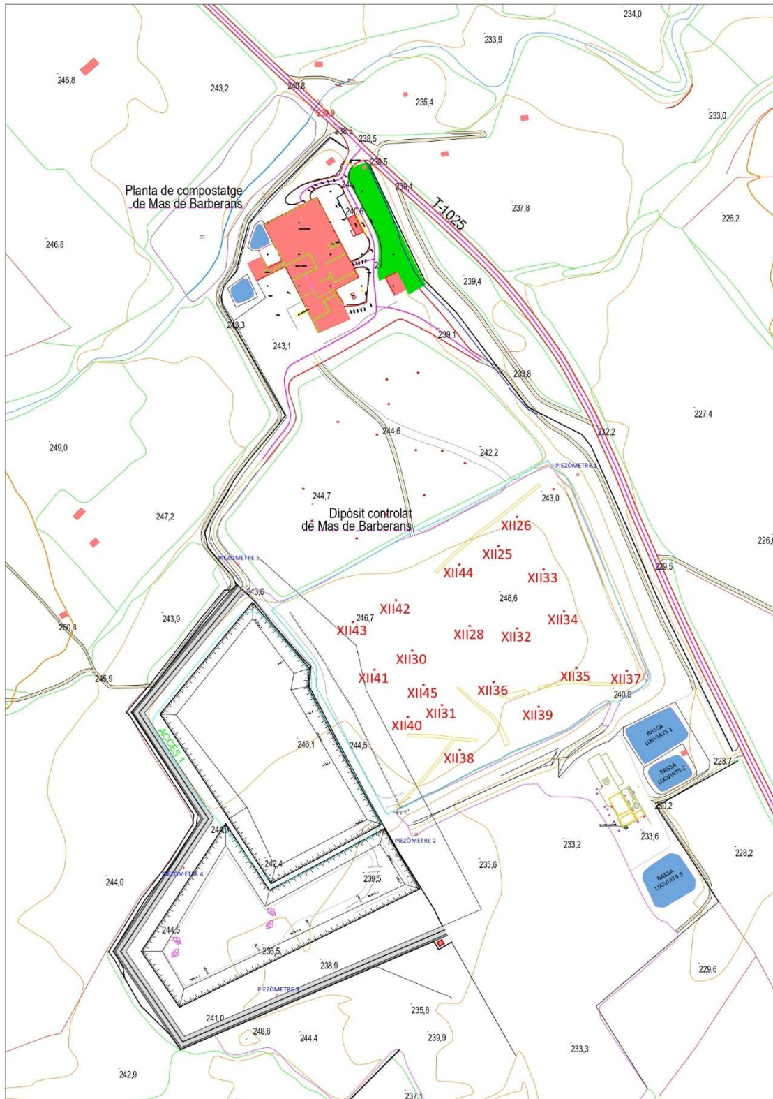
Fig. 2.- Plànol de la xarxa de desgasificació de la fase II del Dipòsit Controlat de Residus de Mas de Barberans (xemeneies actuals).
