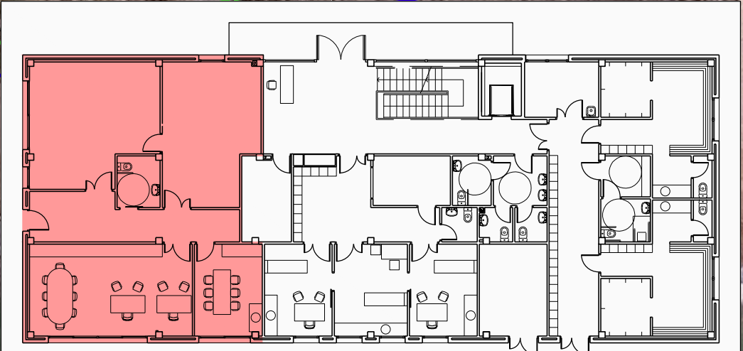
Edifici 1. Planta Baixa. E:1/250
