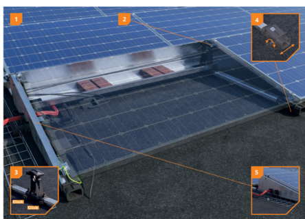
Fig 3. Imatge de la fixació de l'estructura a la coberta de l'edifici
