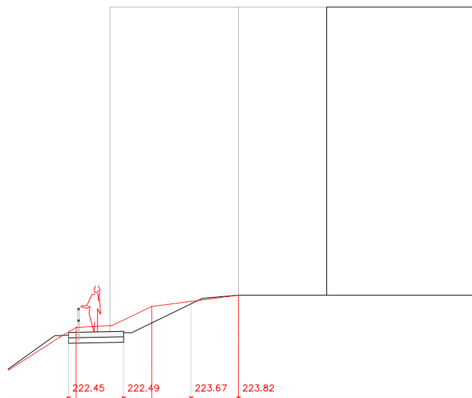
SECCIÓ TRANSVERSAL 1 E: 1/200
