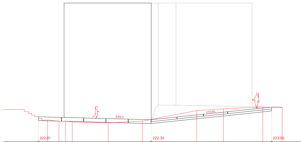
SECCIÓ LONGITUDINAL S1 E: 1/250
