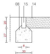
D07 PAVIMENT DE SAULÓ AMB VORADA P3
