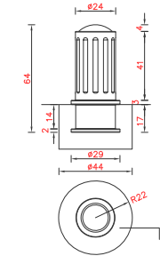
D16 PILONA VIA JULIA
