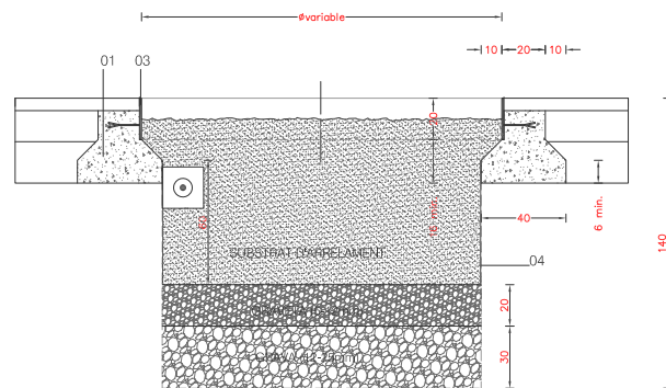
SECCIÓ
