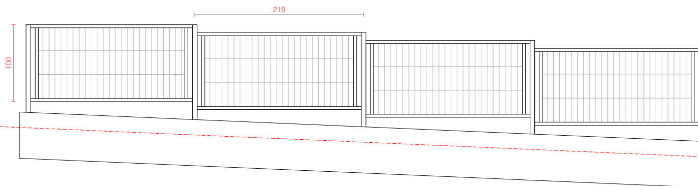
DETALL ALÇAT TANCA E: 1/50
