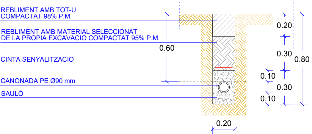
RASA TIPUS EN TERRENY NATURAL
