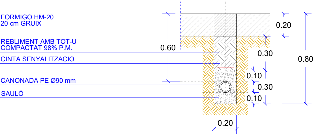
RASA TIPUS EN PAVIMENT ASFÀLTIC
