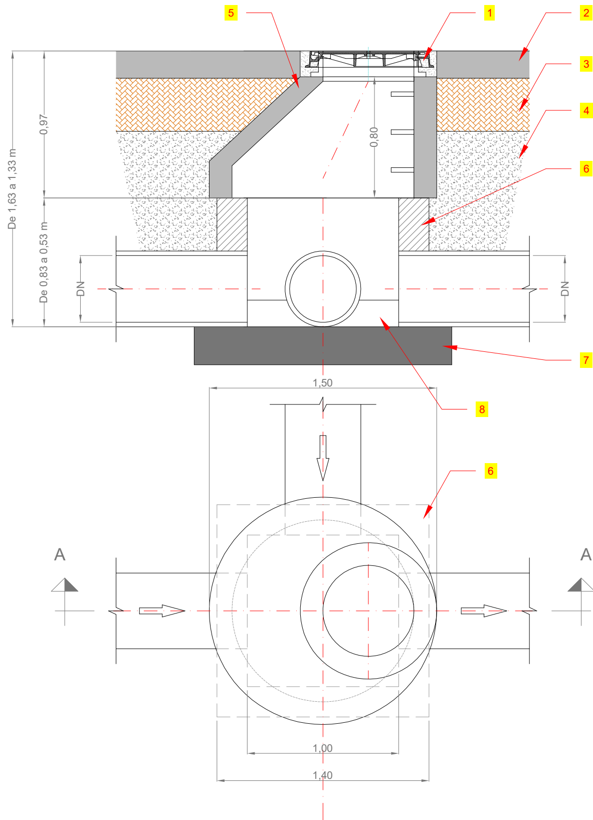
DETALL TIPUS POU DE REGISTRE Esc.: 1/25
