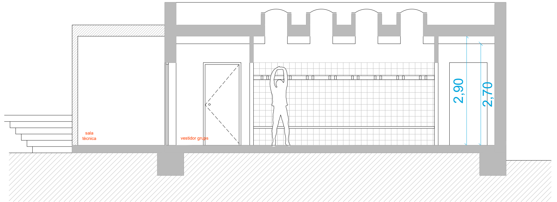
SECCIÓ 1/60
