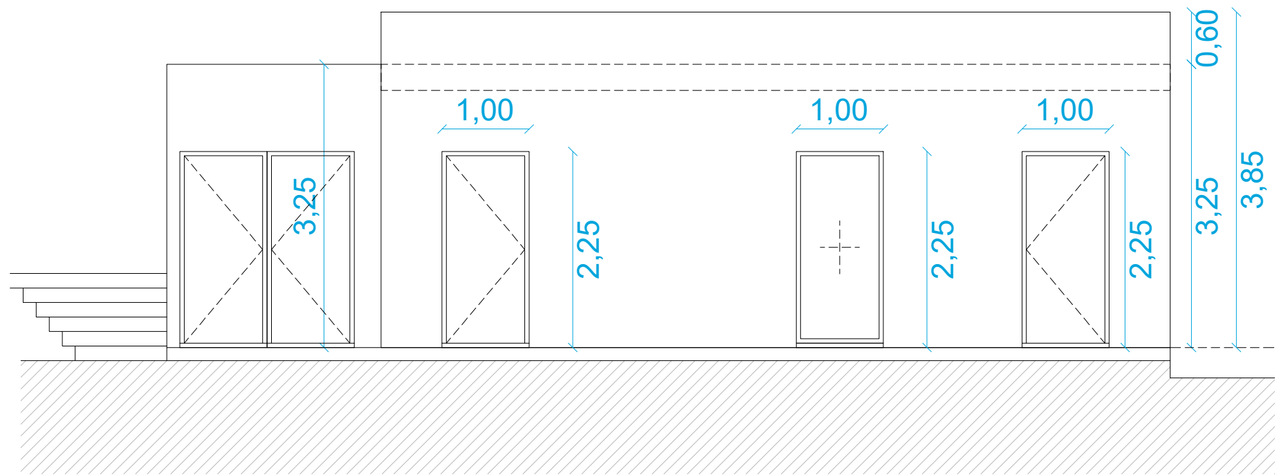
ALÇAT 1/60
