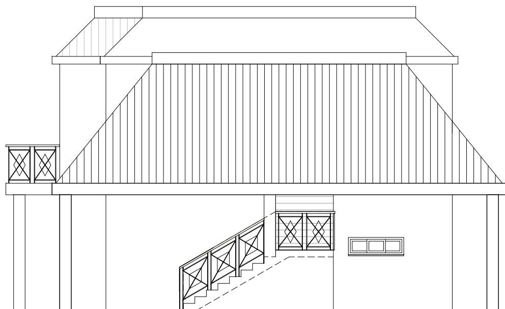
ALÇAT FAÇANA EST
