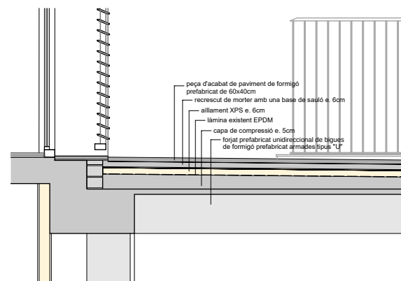
SECCIÓ A-A' _ DETALLS ESTAT ACTUAL _ 1/50
