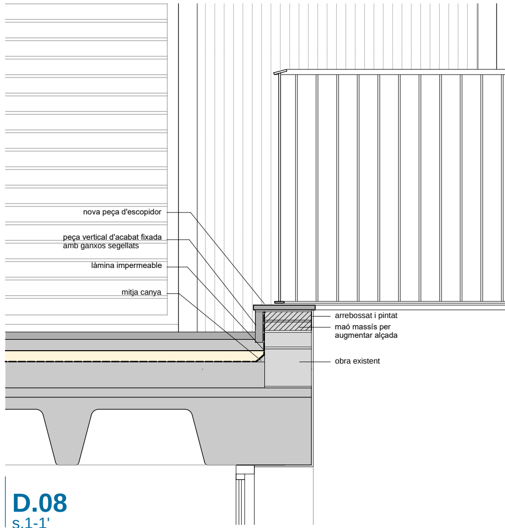
D.08' s.1-1'
