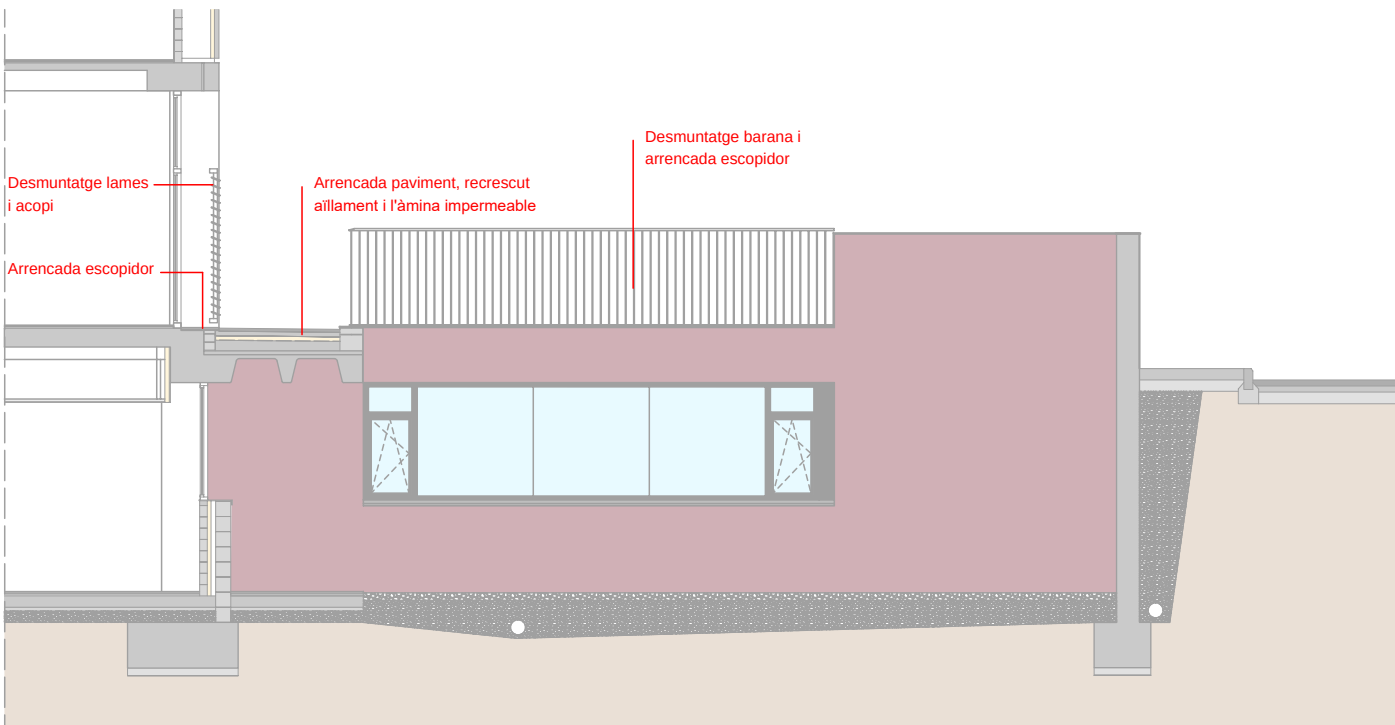
SECCIÓ B-B'_ ELEMENTS A RETIRAR _1/100
