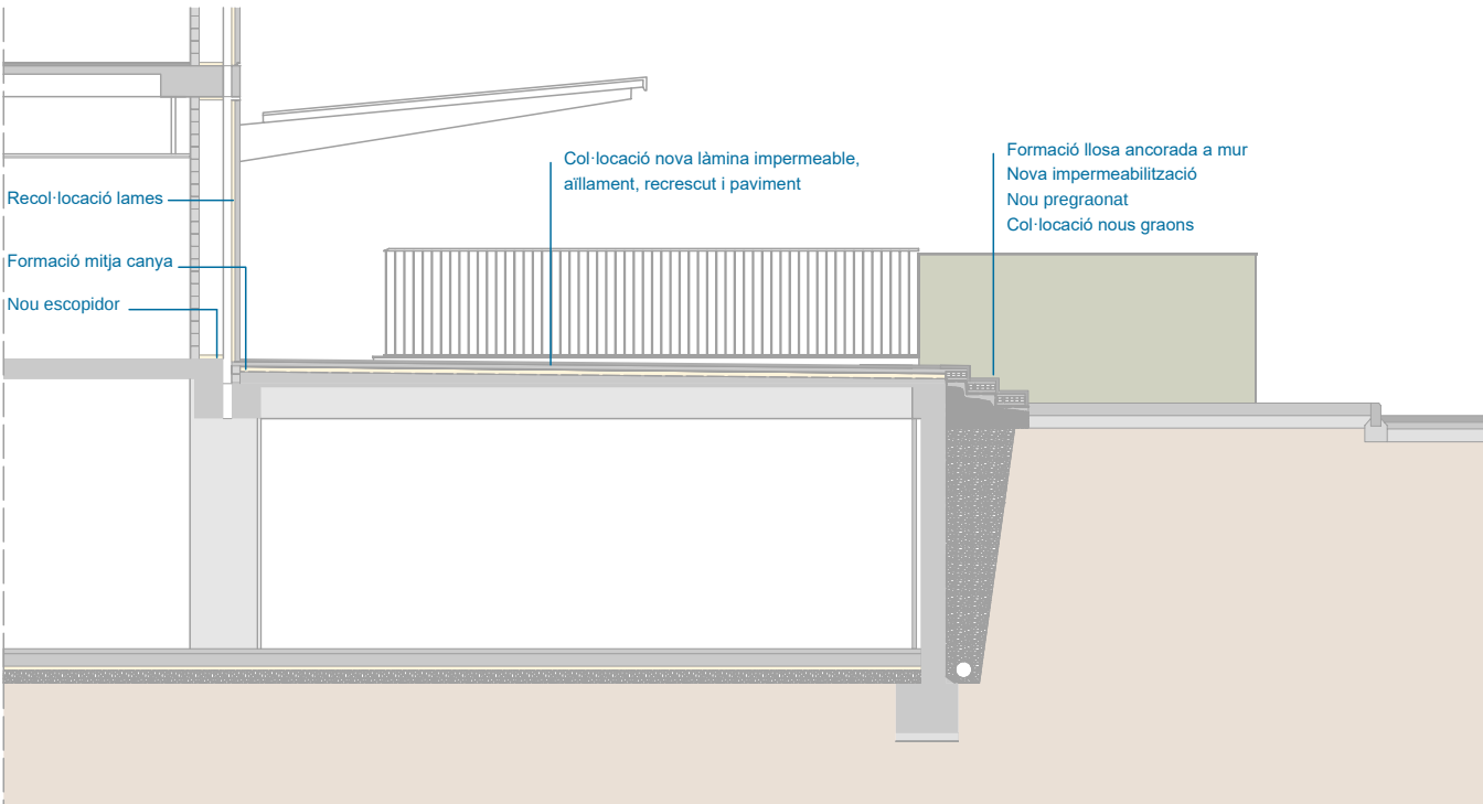
SECCIÓ A-A'_ INTERVENCIONS _1/100
