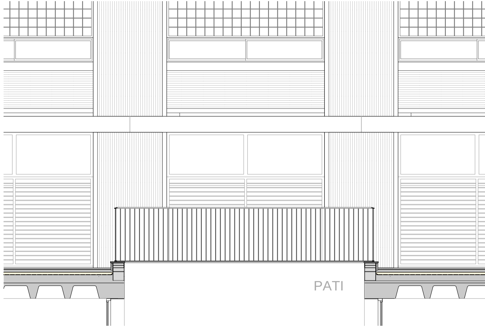
SECCIÓ 1-1'_ PROPOSTA _1/50
