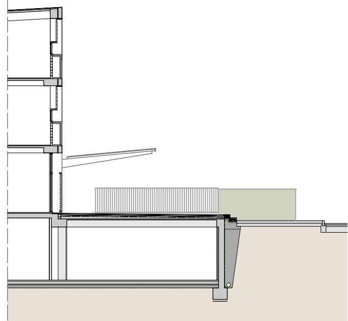
SECCIÓ A-A' _ ESTAT ACTUAL _ 1/200
