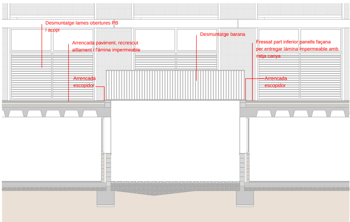
SECCIÓ 1-1'_ ELEMENTS A RETIRAR _1/100
