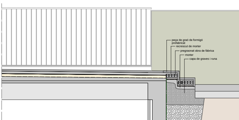
SECCIÓ B-B' _ ESTAT ACTUAL _ 1/200
