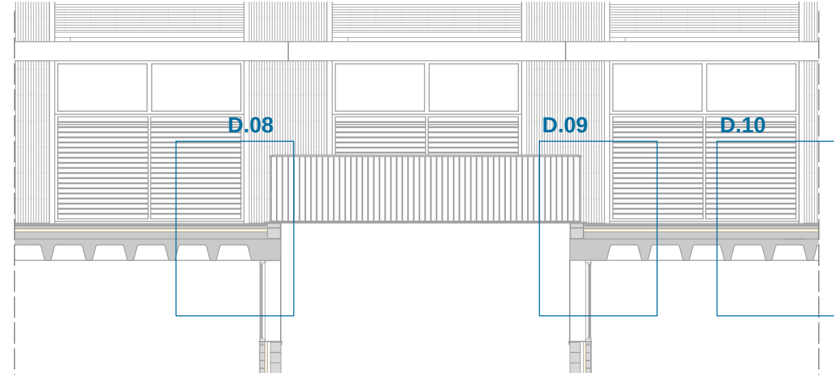
SECCIÓ 1-1'_ PROPOSTA _ 1/100
