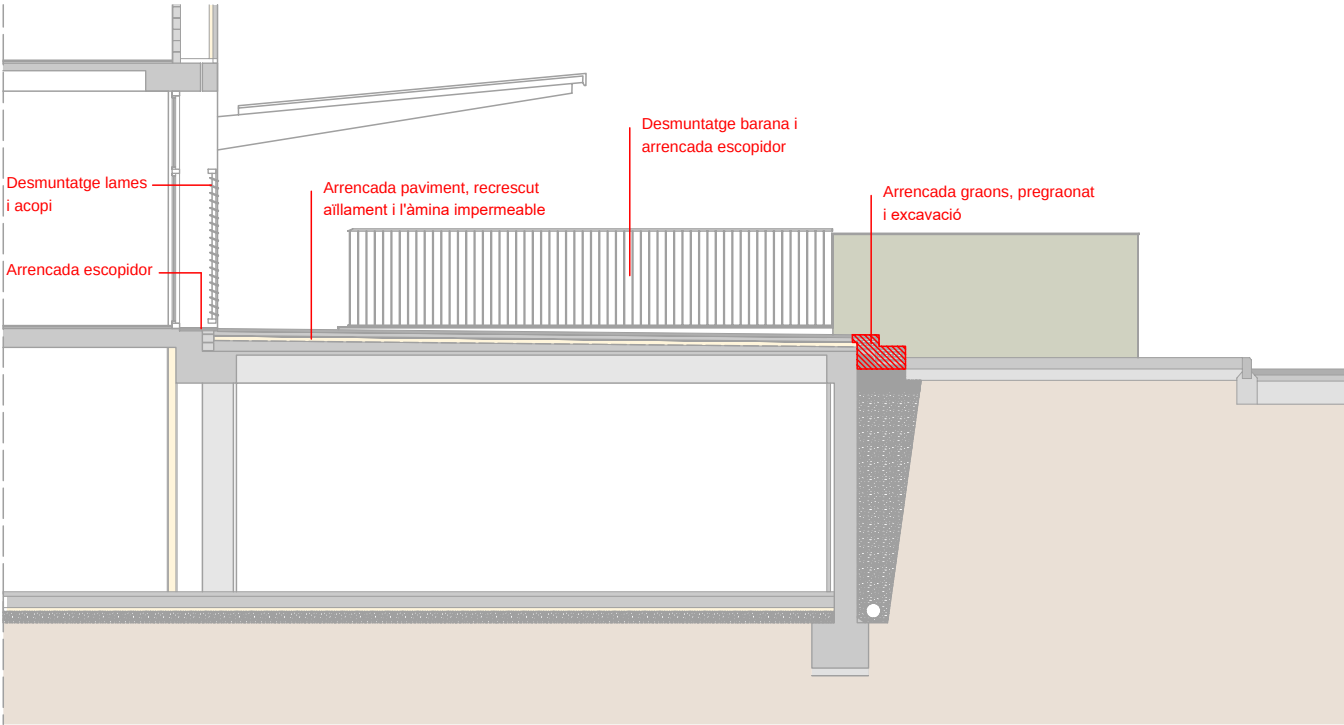
SECCIÓ A-A'_ ELEMENTS A RETIRAR _1/100
