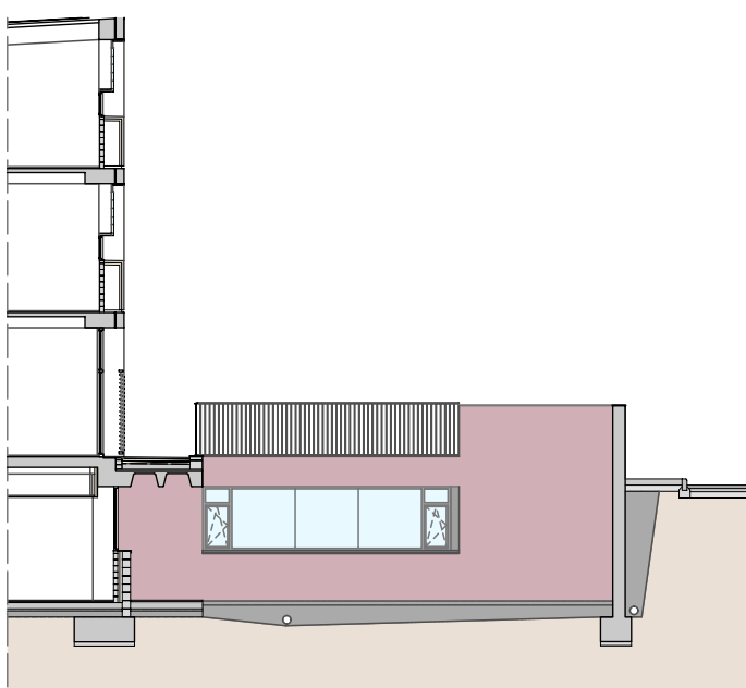
SECCIÓ B-B' _ ESTAT ACTUAL _ 1/200
