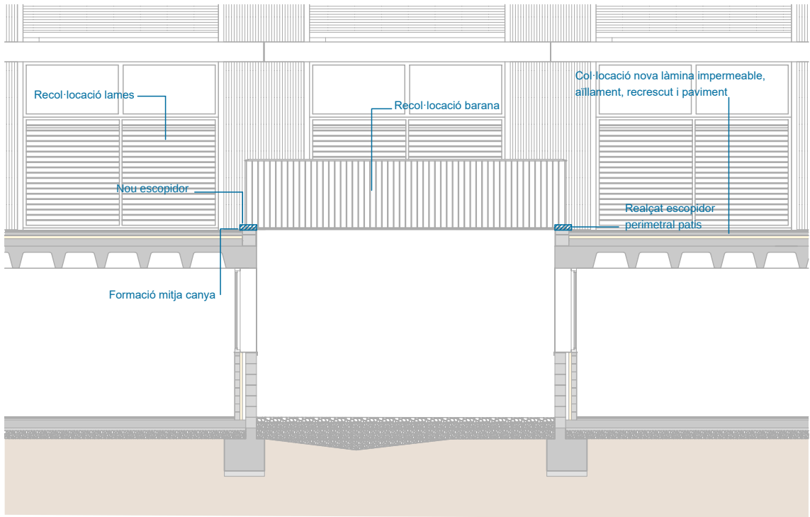
SECCIÓ 1-1'_ INTERVENCIONS _1/100
