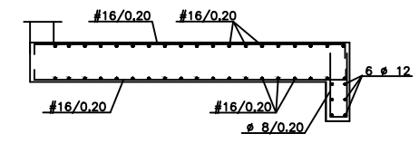
ALÇAT SOLERA I RASTRELL IN SITU
