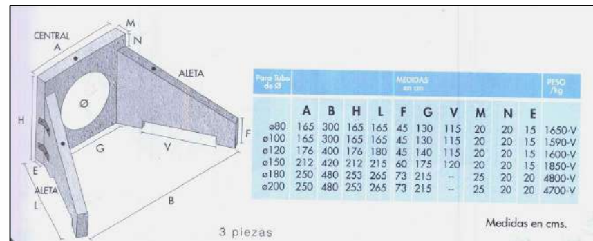
DETALL EMBOCADURA PREFABRICADA PER OD SEGONS Ø
