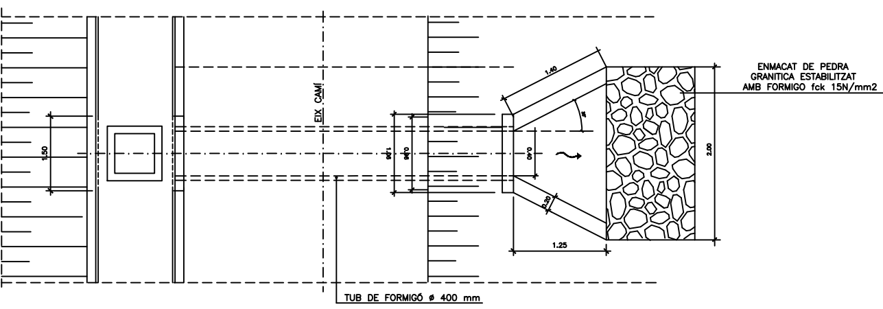
PLANTA
