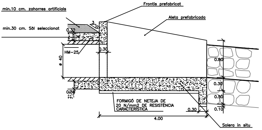
ALÇAT ALETA I SOLERA
