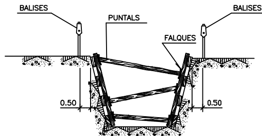
AMPLADA < 3.00m.
