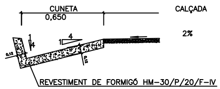
CUNETA REVESTIDA
