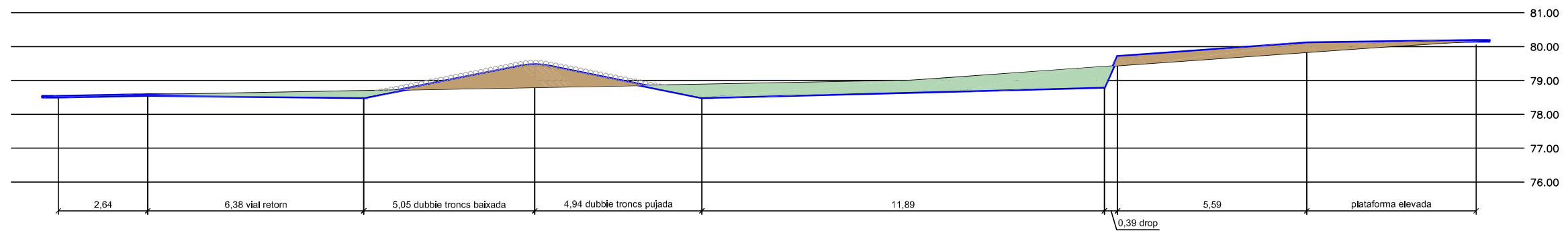
ST7 - SECCIÓ TRANSVERSAL
