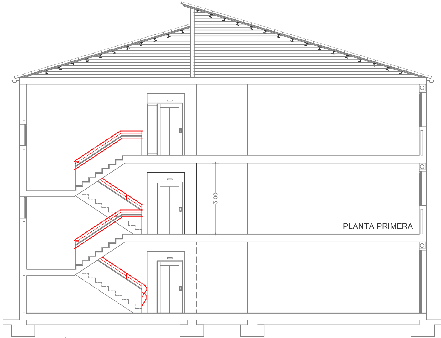
SECCIÓ TRANSVERSAL
