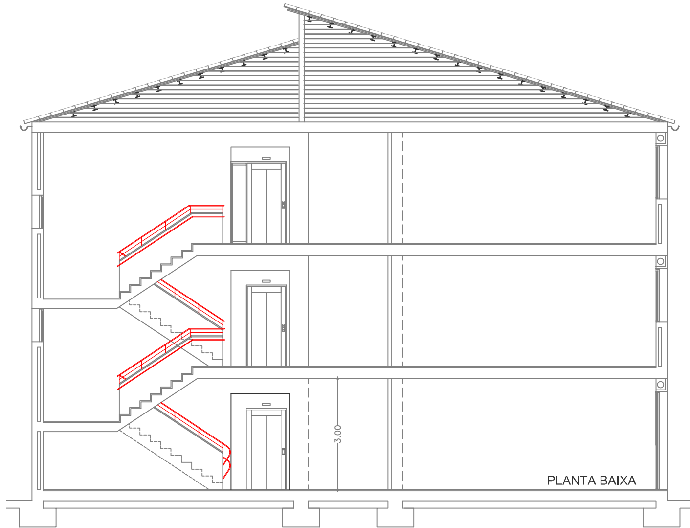
SECCIÓ TRANSVERSAL
