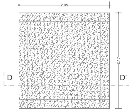
Llosa fonamentació
