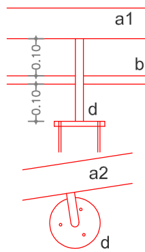
SECCIÓ TRANSVERSAL
