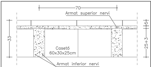
Detall del sostre reticular existent tipus DOLMEN
