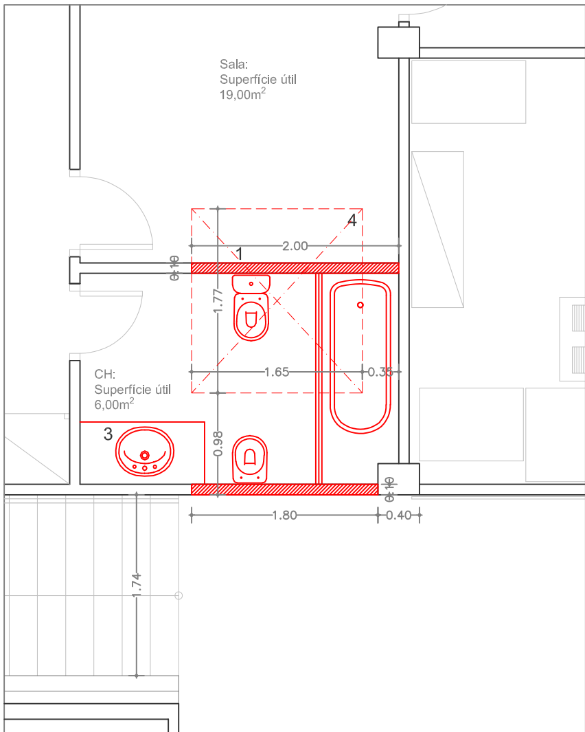
PLANTA BAIXA
