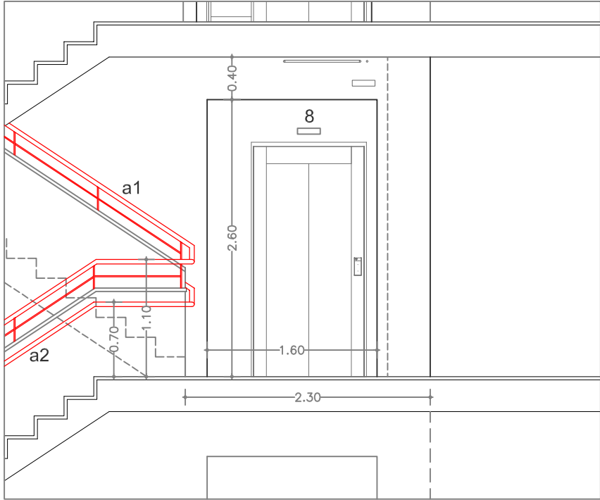
ALÇAT PLANTA PRIMERA
