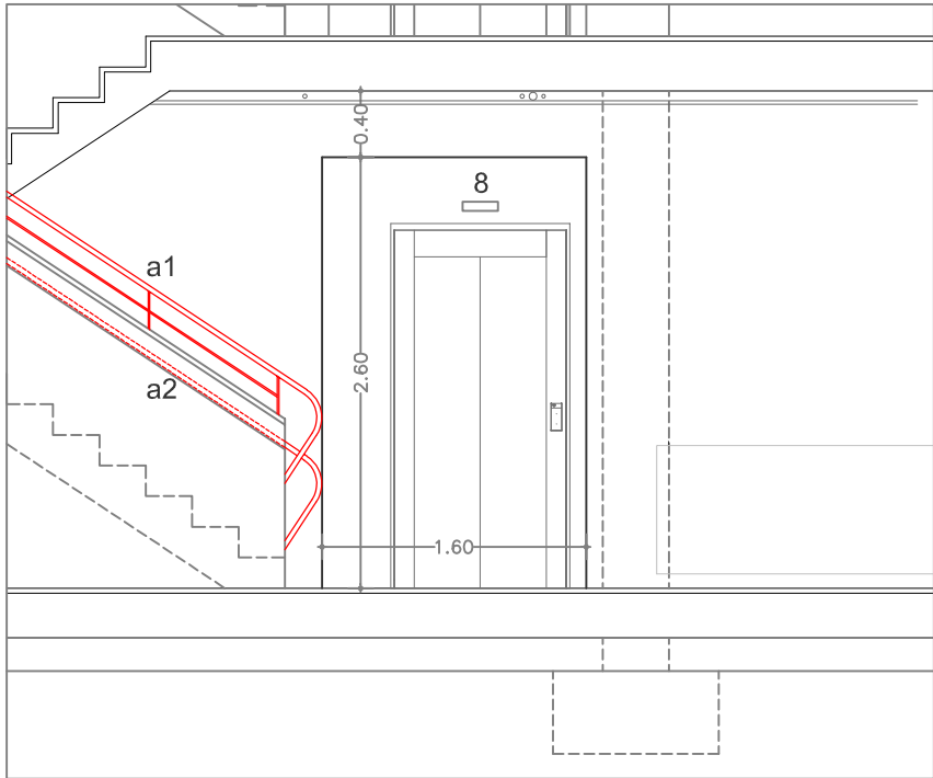
ALÇAT PLANTA BAIXA
