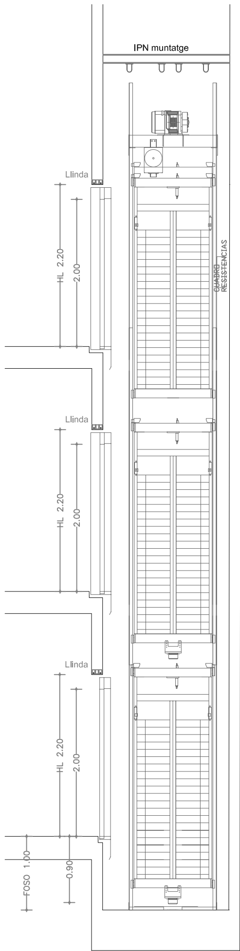
ALÇAT CONTRAPÈS
