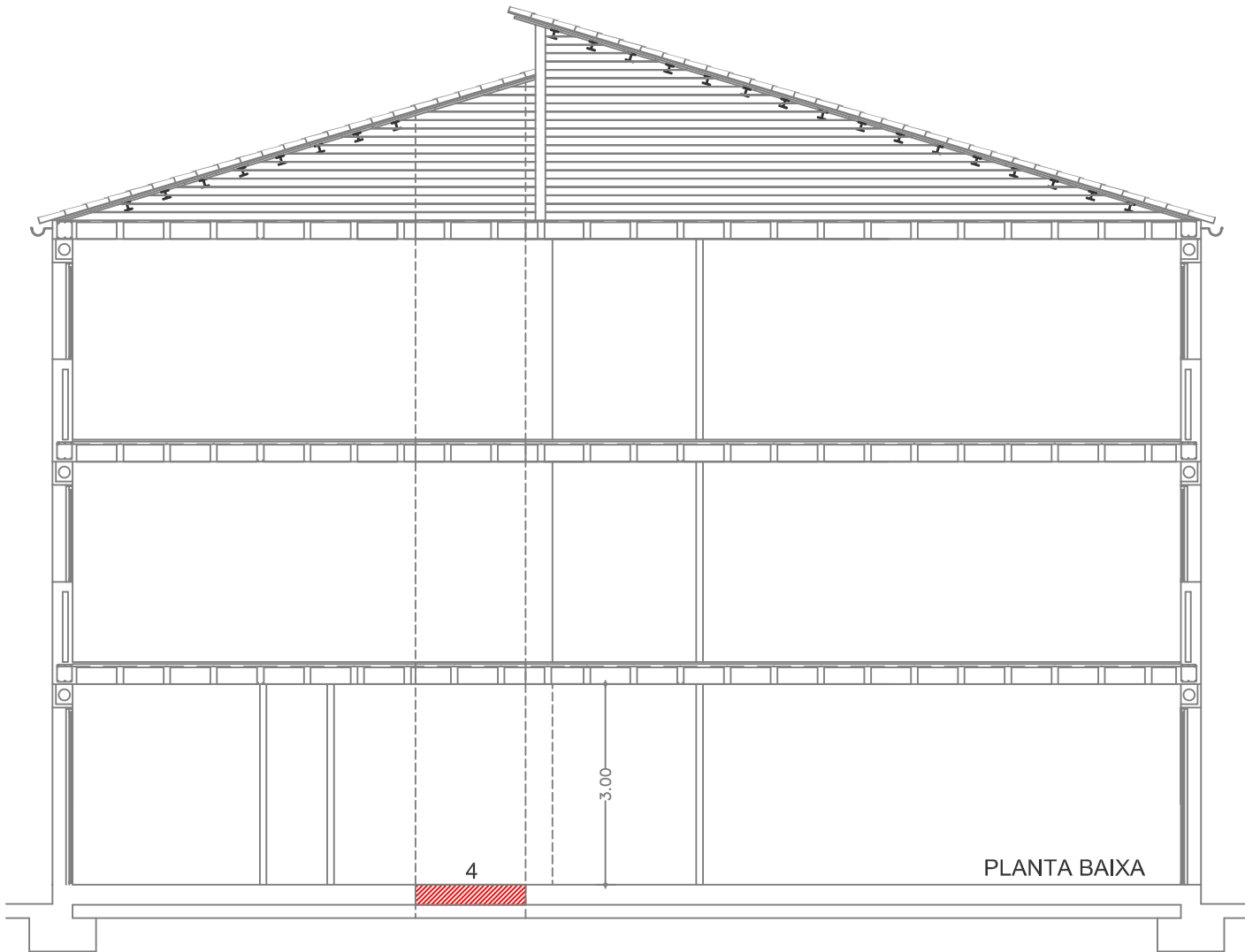
SECCIÓ TRANSVERSAL
