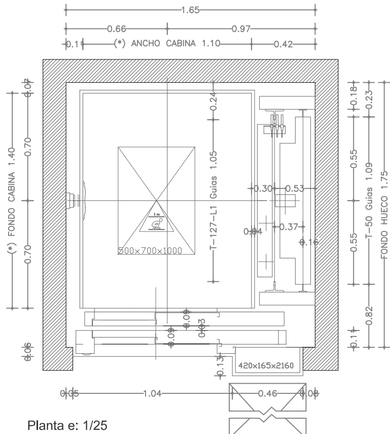
Planta e: 1/25
