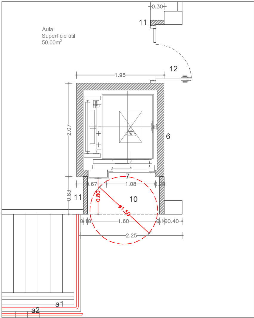
PLANTA SEGONA
