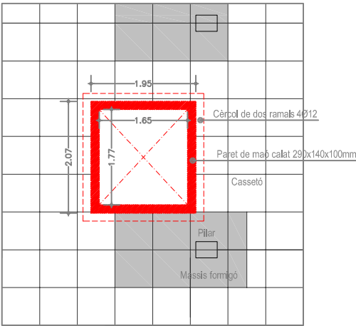
Detall del sostre reticular existent tipus DOLMEN
