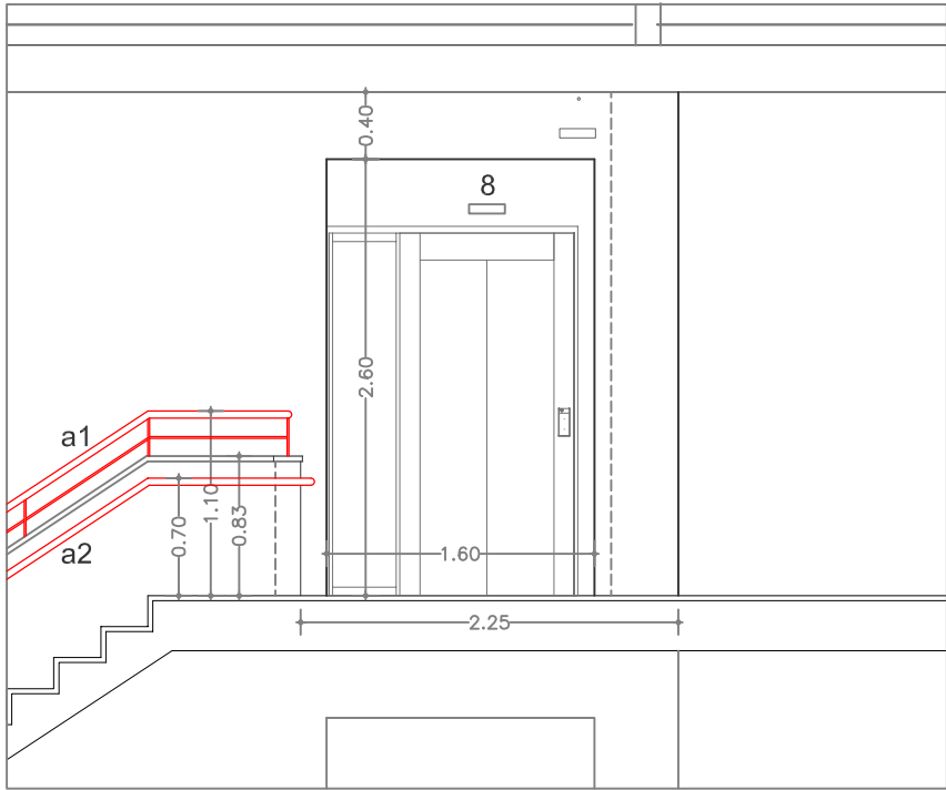
ALÇAT PLANTA SEGONA
