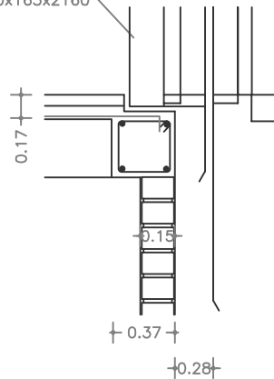
Detall B. e:1/25
