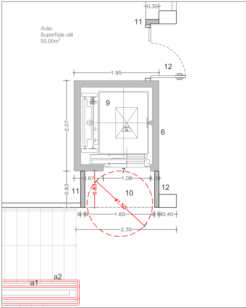
PLANTA PRIMERA
