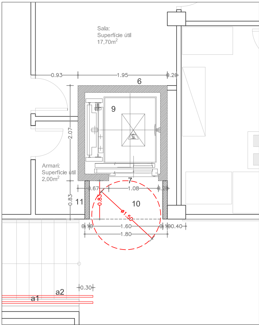
PLANTA BAIXA
