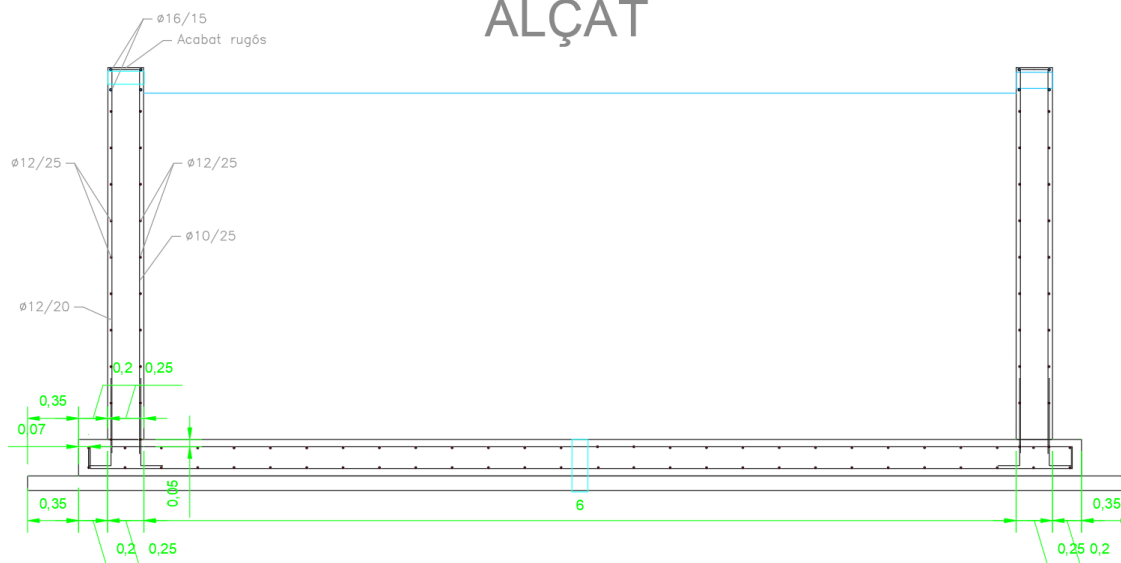
Imatge 27: Esquema de l'armat de les parets del punt d'aigua.
