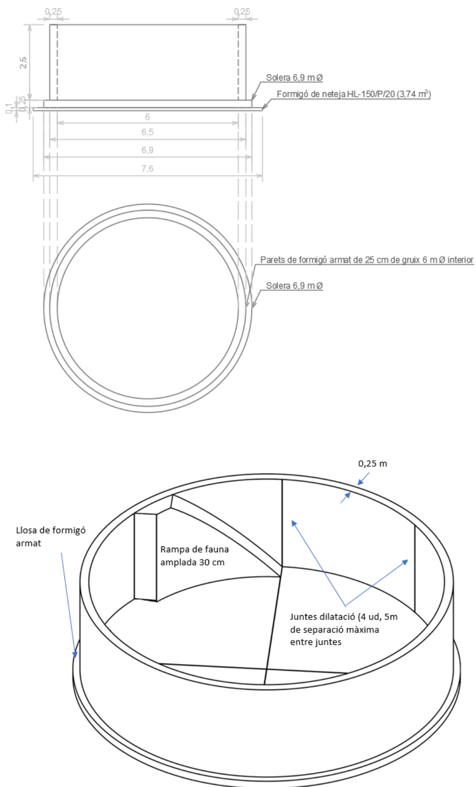
Imatge 22: Esquema del nou punt d'aigua proposat
