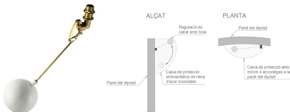
Imatge 31: Automatisme de regulació de cabal i esquema orientatiu de la caixa de protecció.
