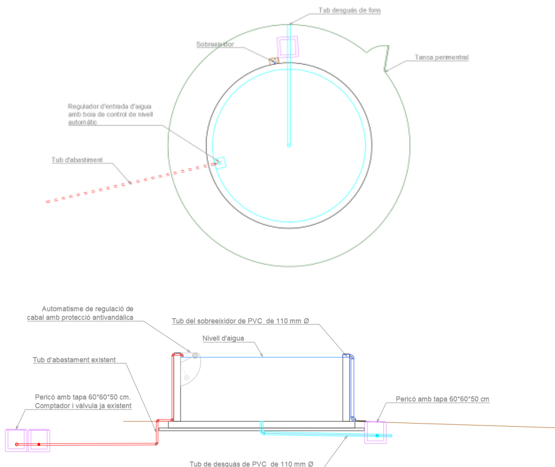
Imatge 33: Elements hidràulics dels punts d'aigua.
