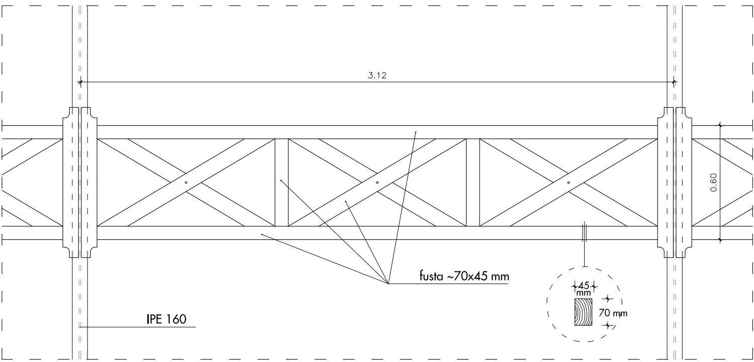
detall 2 - encavallada de fusta longitudinal
