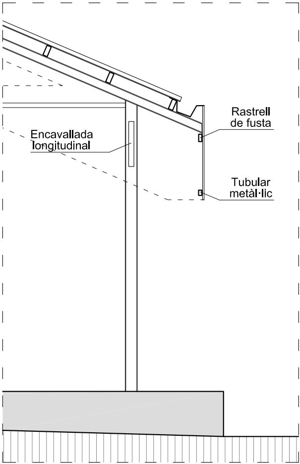
detall 2 - secció encavallada ; e: 1/50
