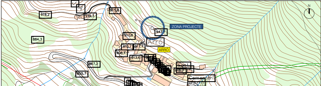
PLÀNOL EMPLAÇAMENT (DIPÒSIT ARRÓ) ESCALA 1/5000
