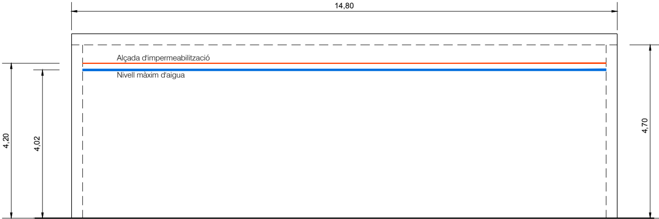
ALÇAT ESCALA 1/100
