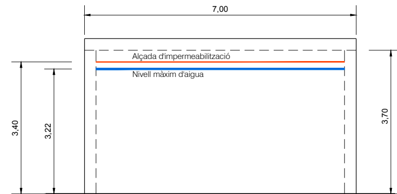
ALÇAT ESCALA 1/100
