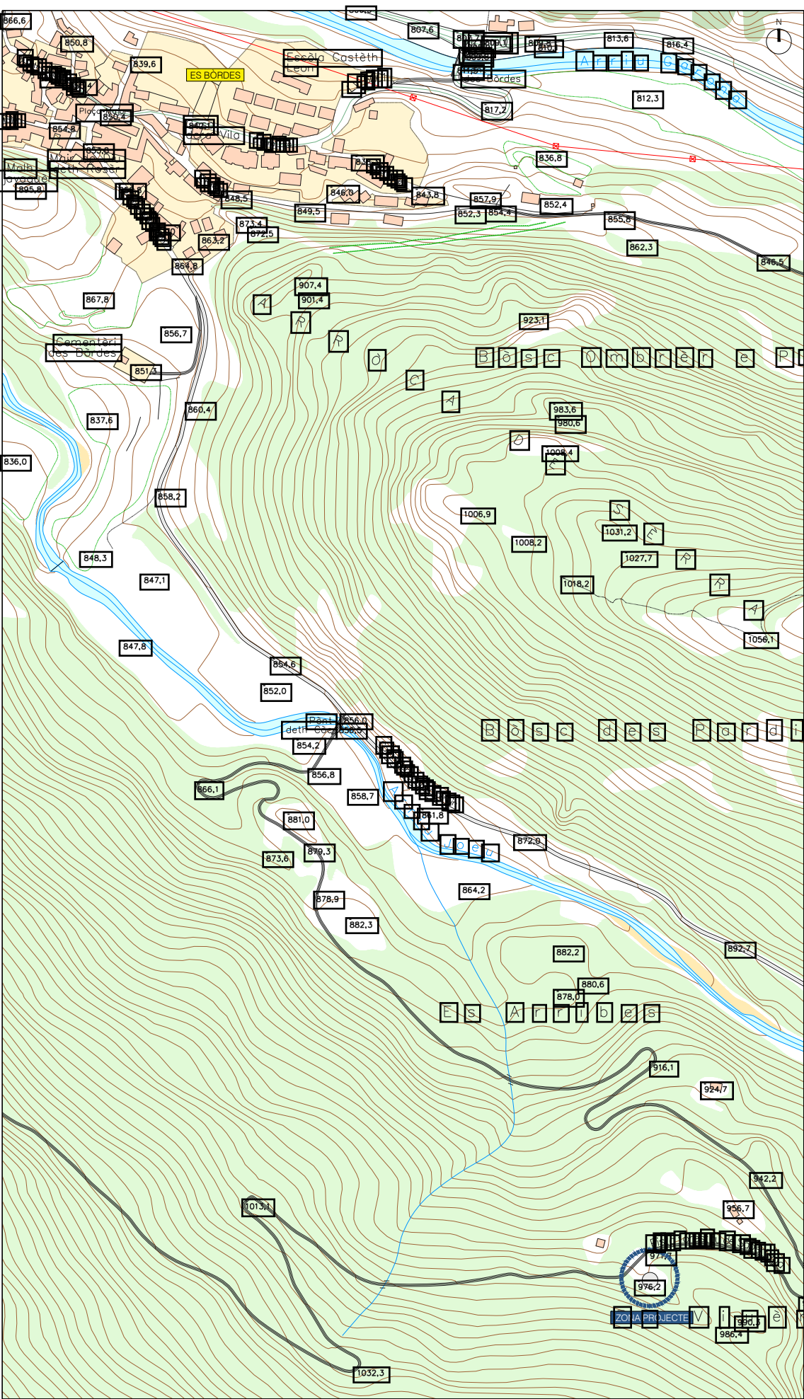
PLÀNOL EMPLAÇAMENT (DIPÒSIT D'ES BÒRDES) ESCALA 1/5000
