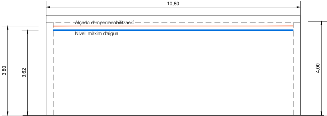
ALÇAT ESCALA 1/100
