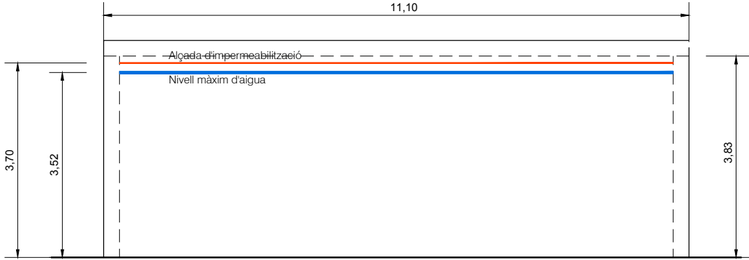
ALÇAT ESCALA 1/100
