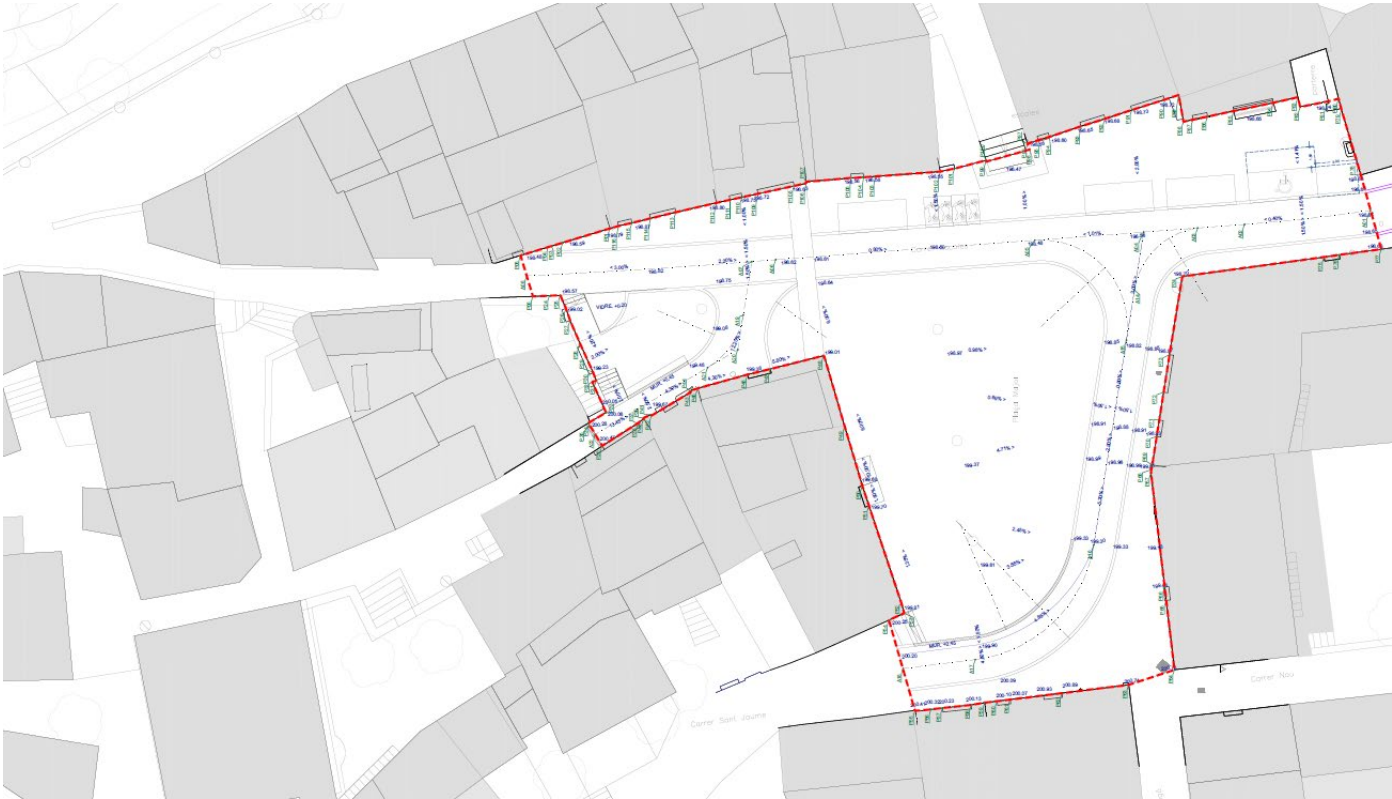
Figura 19. Traçat i replanteig de la plaça Major Font. Elaboració pròpia
