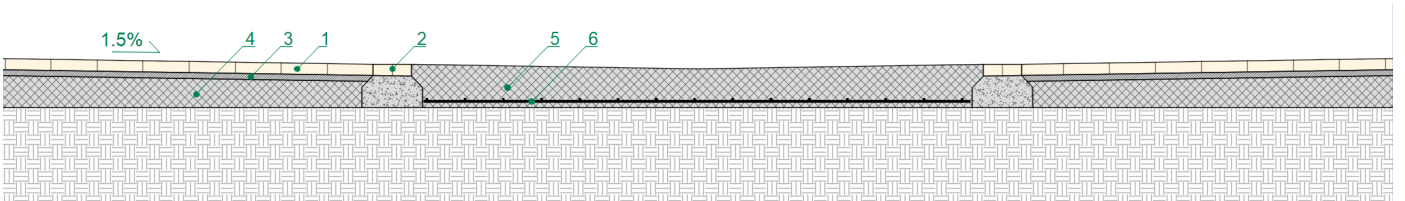
Figura 24. Detall constructiu de proposta de ferm Font. Elaboració pròpia
