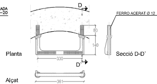
Alçat
