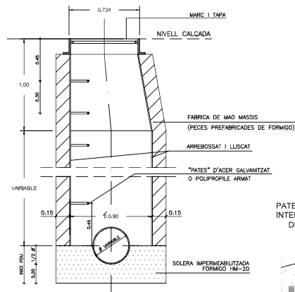
SECCIO C-C
