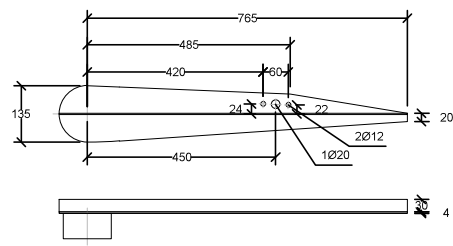
CHAPA CREUETA PLUS BCN PER 1 PROJECTOR CONVENCIONAL
