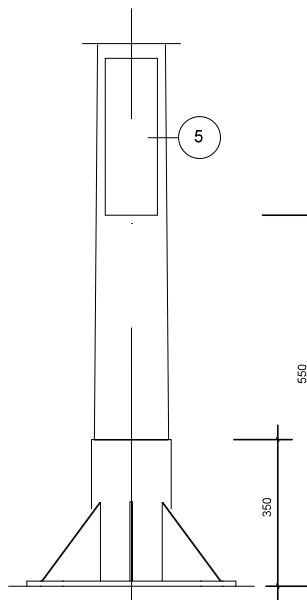
DETALL ALÇAT PLACA E: 1/10
