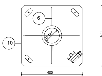
DETALL PLANTA PLACA E: 1/10
