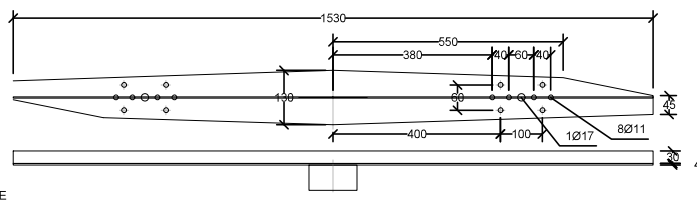
CHAPA CREUETA PLUS BCN PER 2 PROJECTORS CONVENCIONALS
