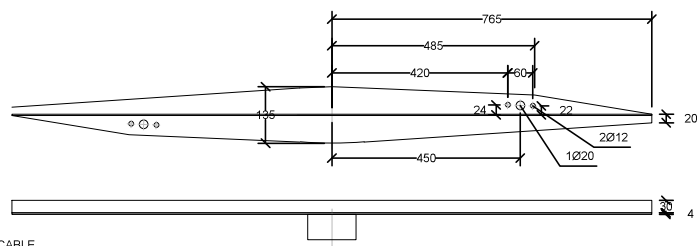
CHAPA CREUETA PLUS BCN PER 2 PROJECTORS CONVENCIONALS
