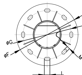
SECCIÓ A-A'
