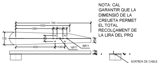
CHAPA CREUETA PLUS BCN PER 1 PROJECTOR PRQ
