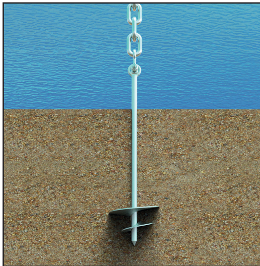
Cordada de boiarins amb anclatge ecològic
