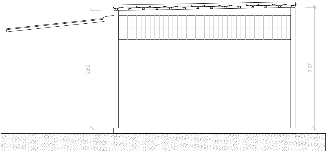
ALÇAT S2 ESCALA 1:50
