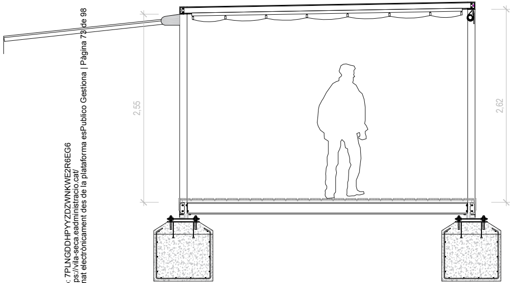
ALÇAT S4 ESCALA 1:50
