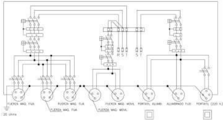
ESQUEMA UNIFILAR DEL CUADRO ELECTRICO DE OBRA
