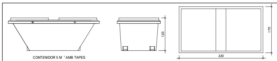
CONTENIDOR 5 M 3 AMB TAPES
