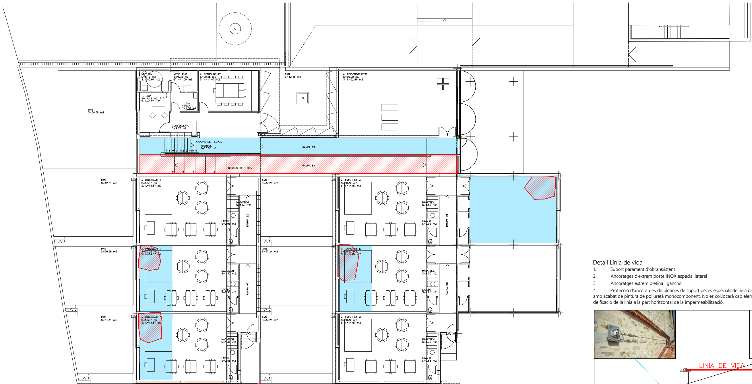
Planta defectes interior E: 1/200
