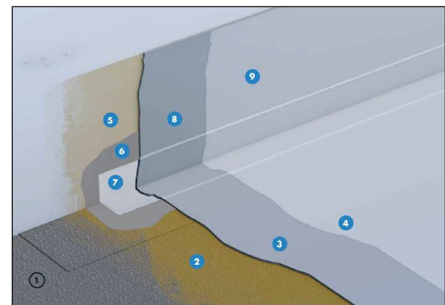
DETALL CAPES IMPERMEABILITZACIÓ
