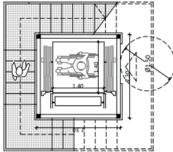
PLANTA BAIXA. Escala i ascensor E: 1/50
