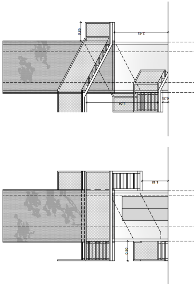
ALÇAT NORD-EST. Escala i ascensor E: 1/50
