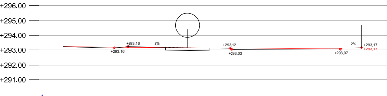
SECCIÓ 10 E 1:250
