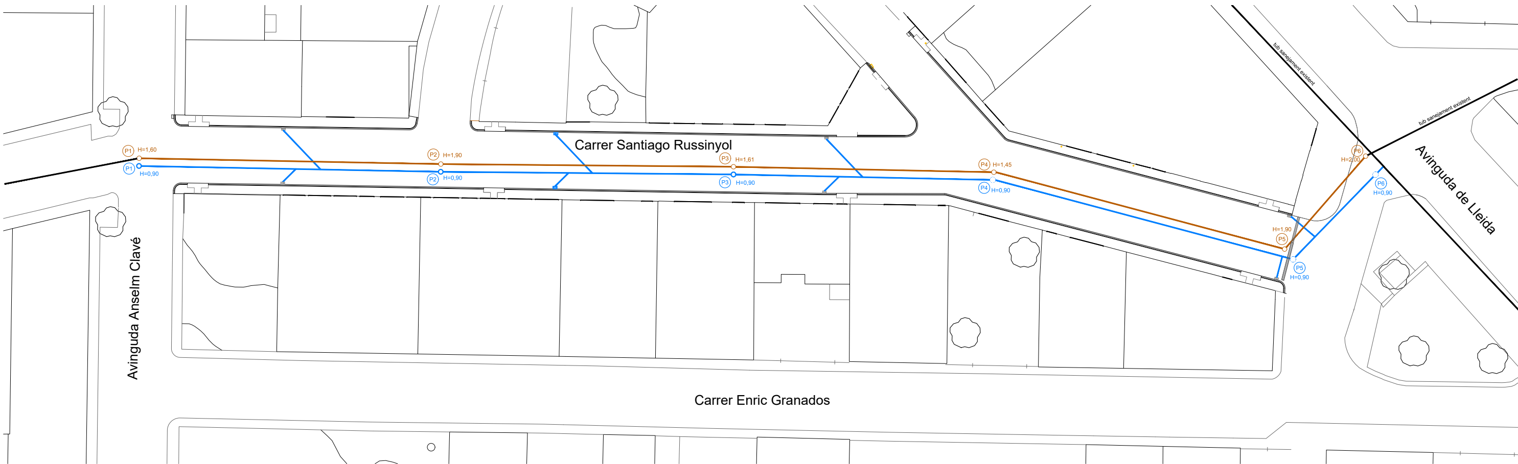
PLANTA INSTAL·LACIÓ - XARXA DE SANEJAMENT E1:500
