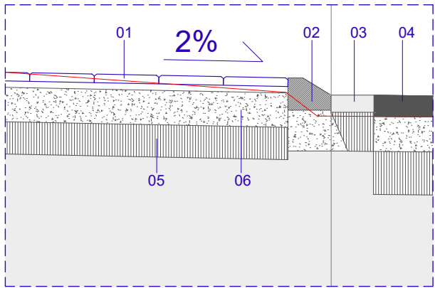
DETALL 01 E 1:25
