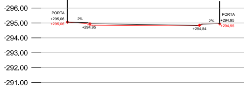
SECCIÓ 3 E 1:250
