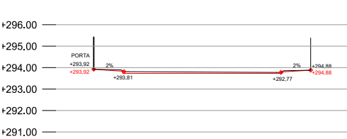
SECCIÓ 7 E 1:250
