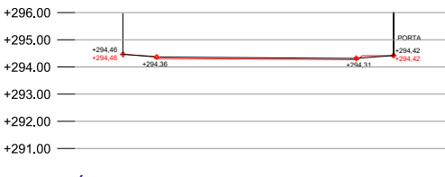
SECCIÓ 5 E 1:250
