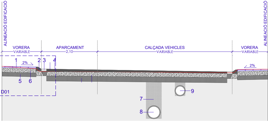
DETALL SECCIÓ CONSTRUCTIVA E 1:75
