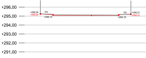
SECCIÓ 2 E 1:250
