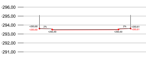
SECCIÓ 8 E 1:250
