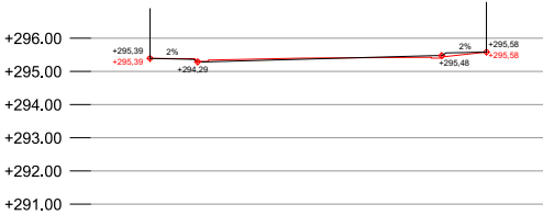
SECCIÓ 1 E 1:250
