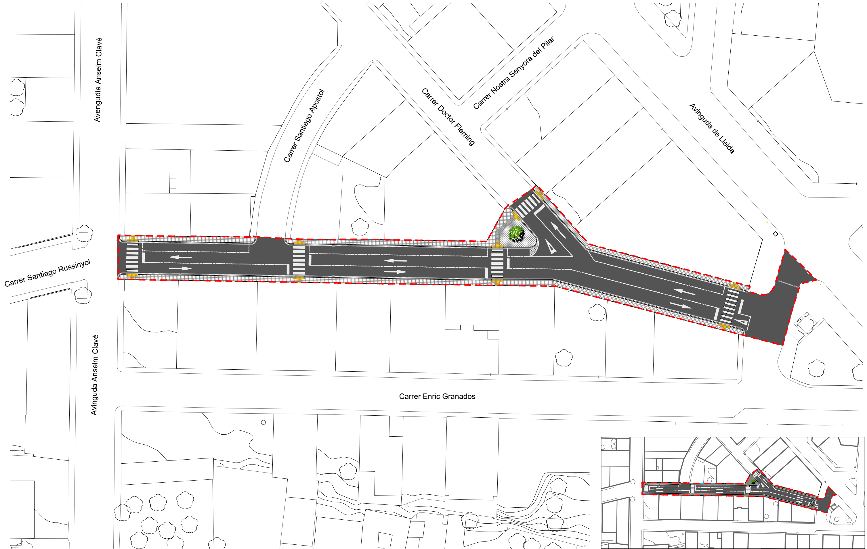
PROPOSTA - EMPLAÇAMENT E1:500
