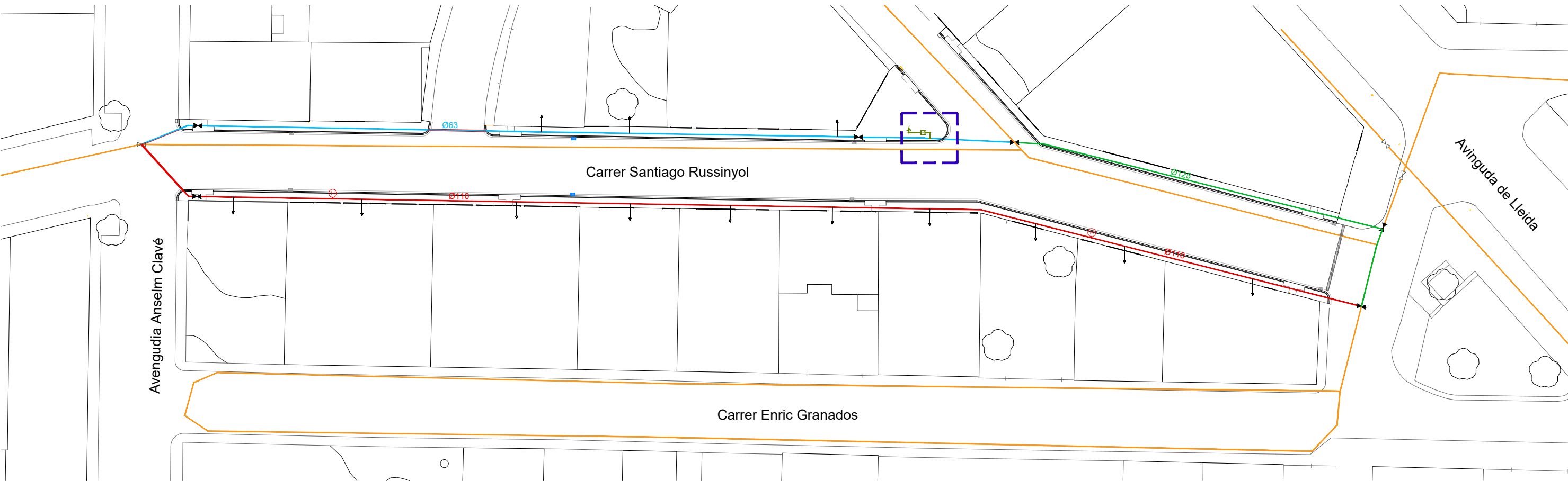
PLANTA INSTAL·LACIÓ - XARXA D'AIGUA POTABLE E1:500
