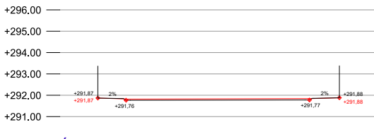
SECCIÓ 16 E 1:250
