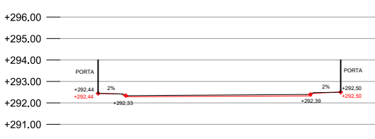
SECCIÓ 14 E 1:250
