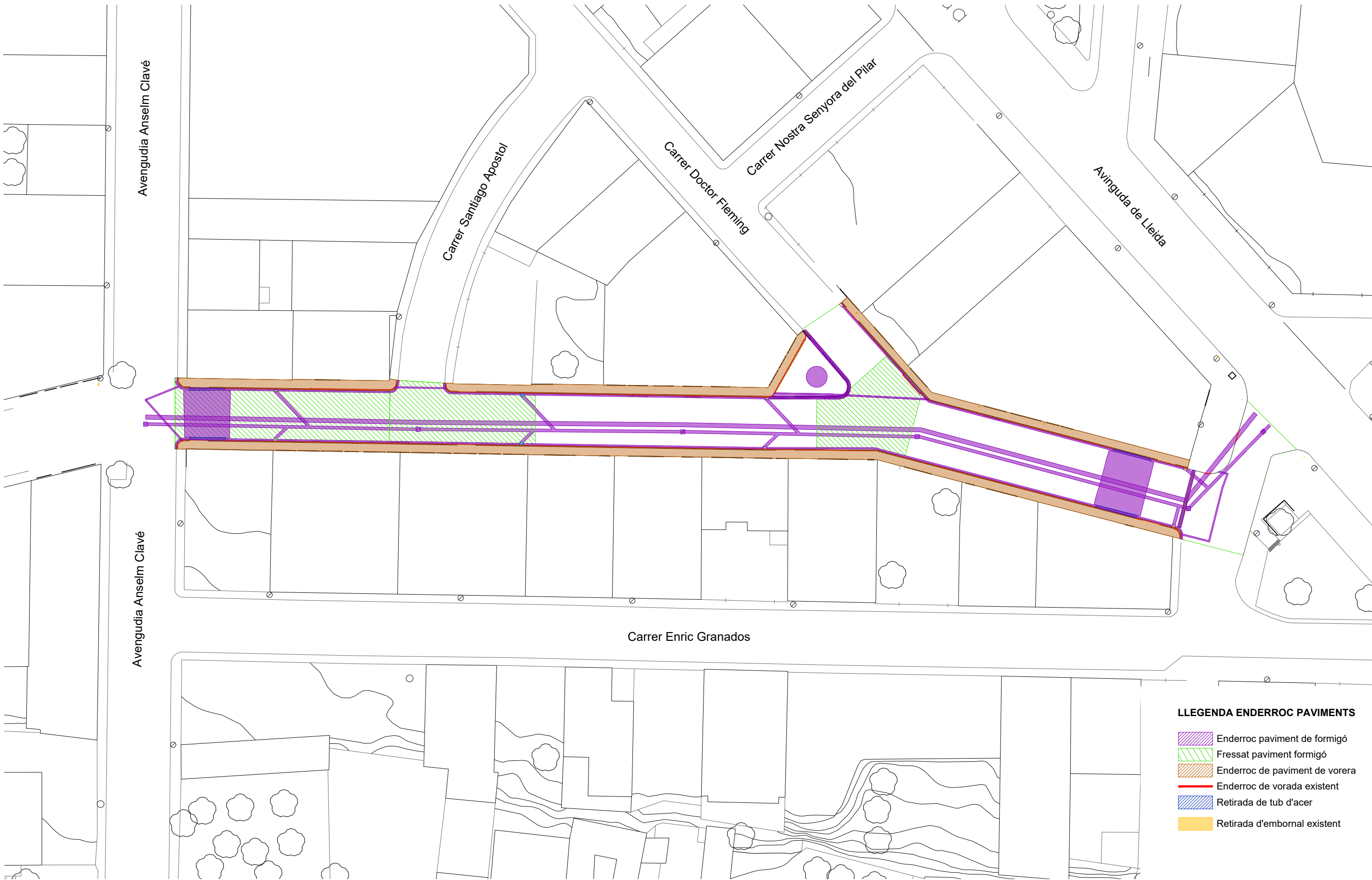
PLANTA ENDERROCS E1:500
