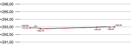
SECCIÓ 12 E 1:250
