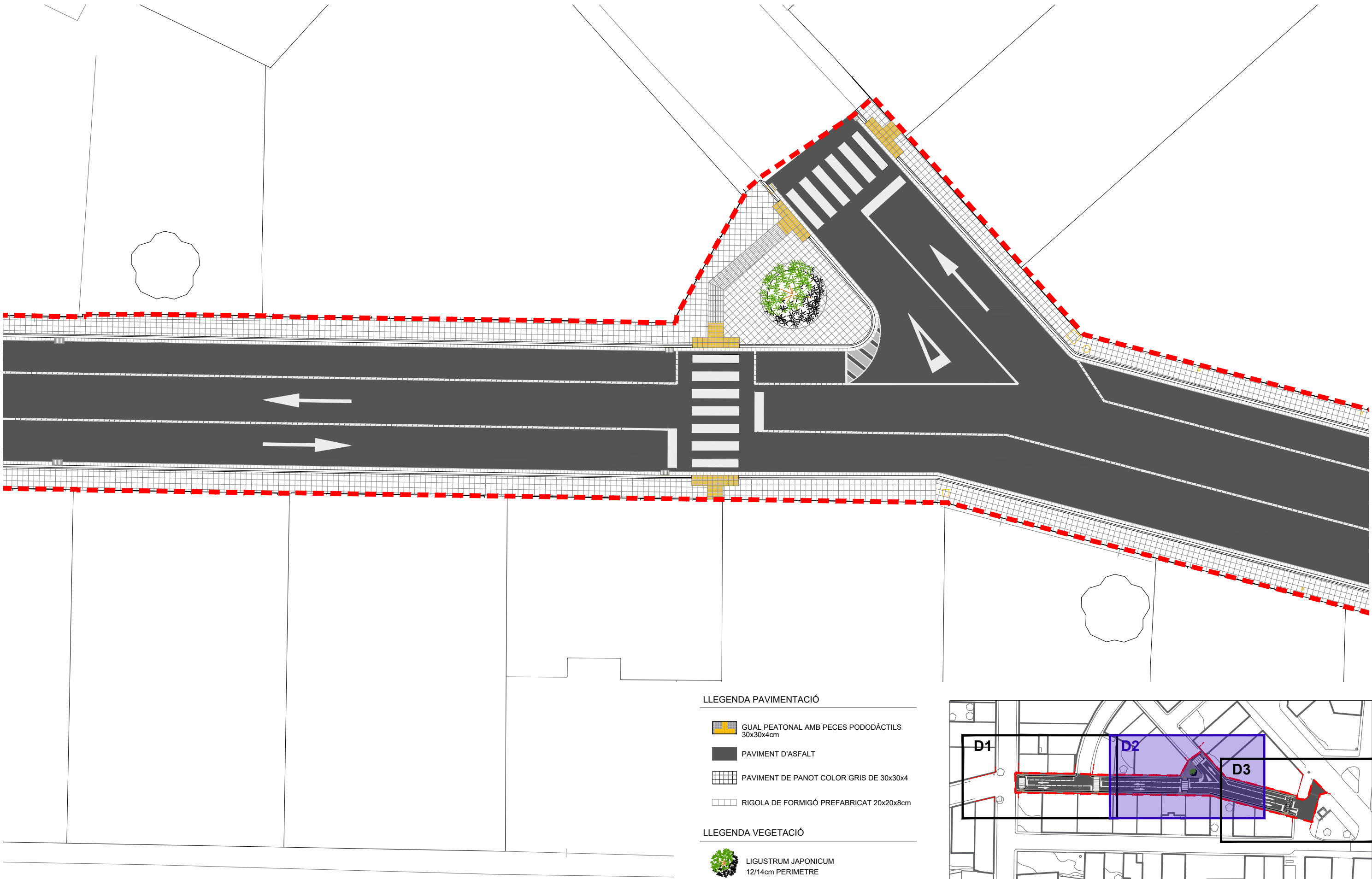
PROPOSTA URBANITZACIÓ -PART D2 - E1:200
