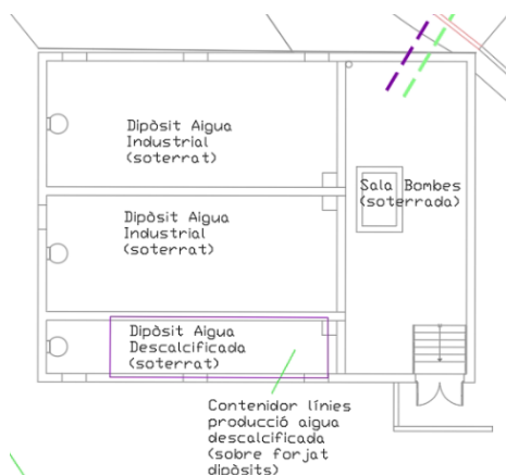
Imatge 5 ubicació contenidor planta descalcificació
