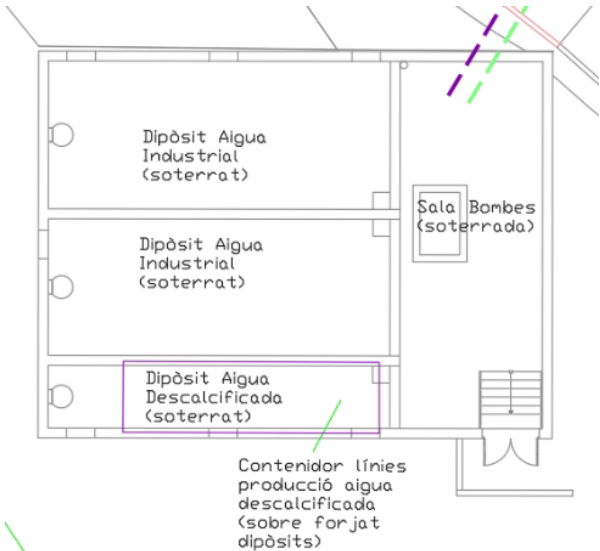
Imatge 3. l'espai previst per a ubicar el contenidor del sistema de descalcificació
