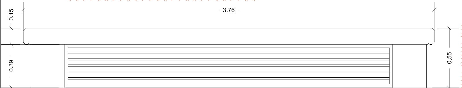
SECCIÓ LONGITUDINAL BANCADA ACCÉS VENTILACIÓ TRAM 3
