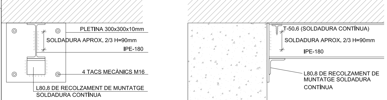
DETALLS SOLDADURES TROBADA PERFILS IPE180 AMB PLETINES ANCORATGE A JÀSSERA FORMIGÓ EXISTENT
