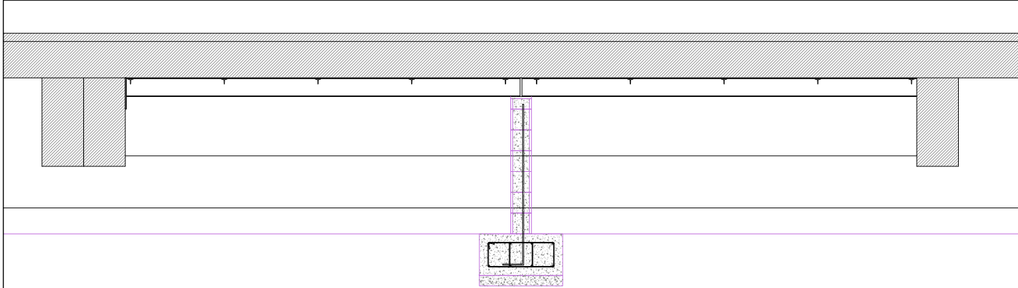
DETALL PLANTA REFORÇ BIGUETES IPE ALS NERVIS MÉS MALMESOS
