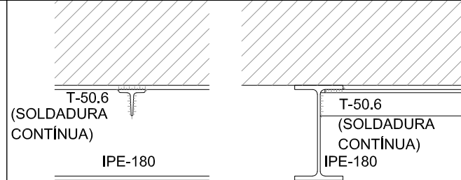
DETALLS SOLDADURES TROBADA PERFILS IPE180 - T50.6
