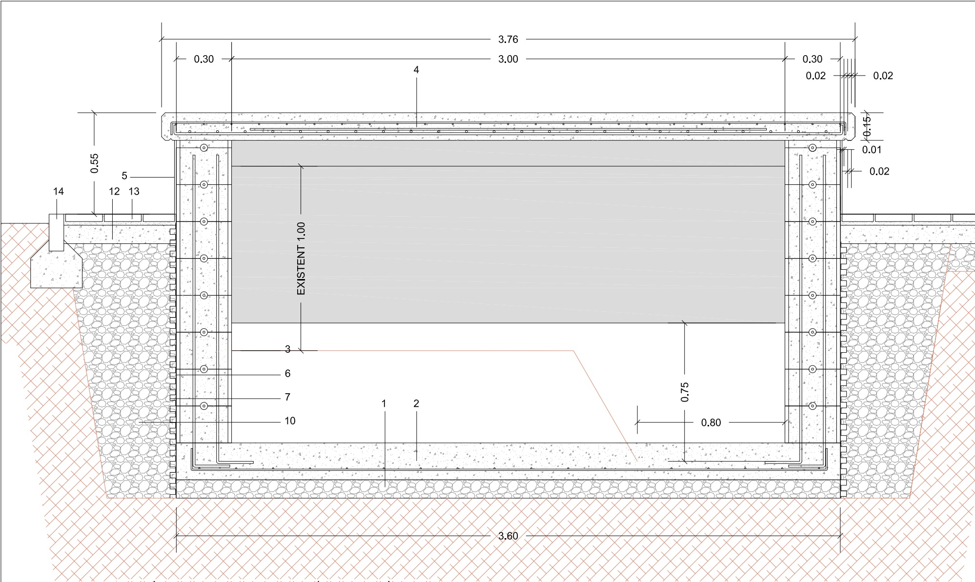
SECCIÓ LONGITUDINAL BANCADA ACCÉS VENTILACIÓ TRAM 3
