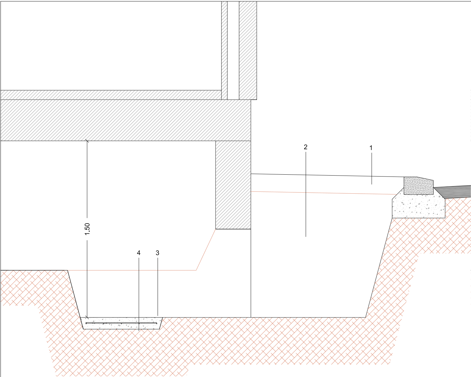
SECCIÓ TRANSVERSAL ACCÉS TRAM 4 - FASE EXECUCIÓ D'OBRA
