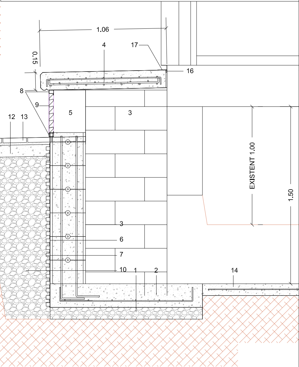
SECCIÓ TRANSVERSAL BANCADA ACCÉS VENTILACIÓ TRAM 3
