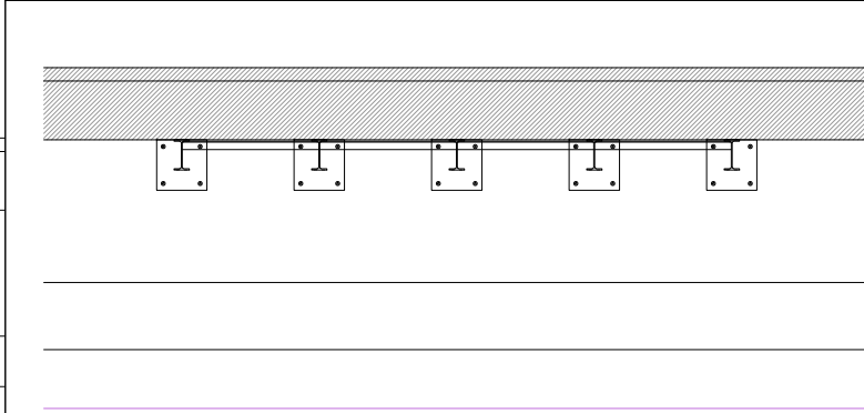
DETALLS SECCIONS REFORÇ BIGUETES IPE ALS NERVIS MÉS MALMESOS
