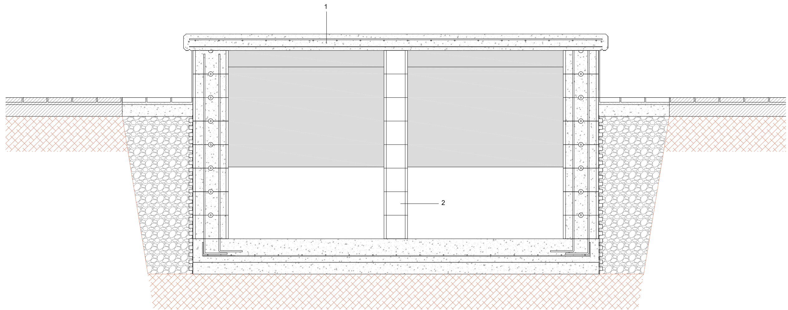
ACCESSOS OBRA TRAM 6 SUD-EST I TRAM 2 - ESTAT ACTUAL
