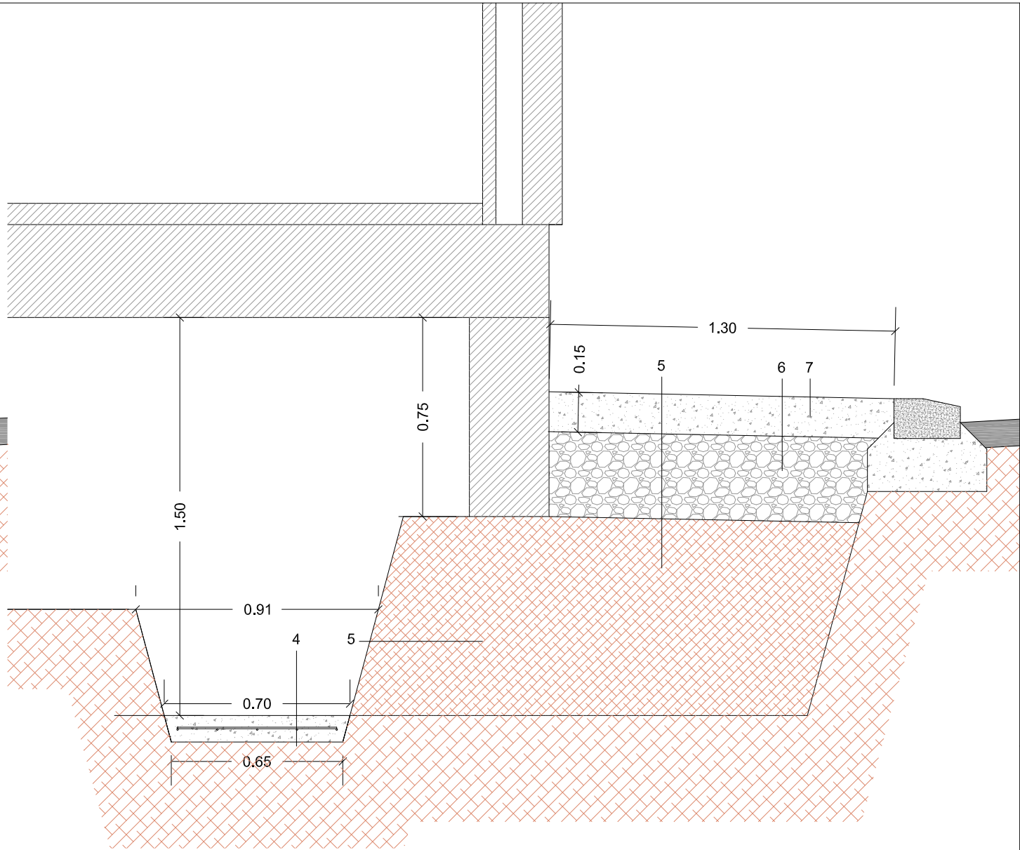
SECCIÓ TRANSVERSAL ACCÉS TRAM 4 - FASE OBRA ACABADA
