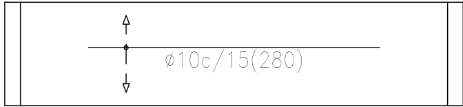
ARMADO LOSAS - REFUERZO INFERIOR
