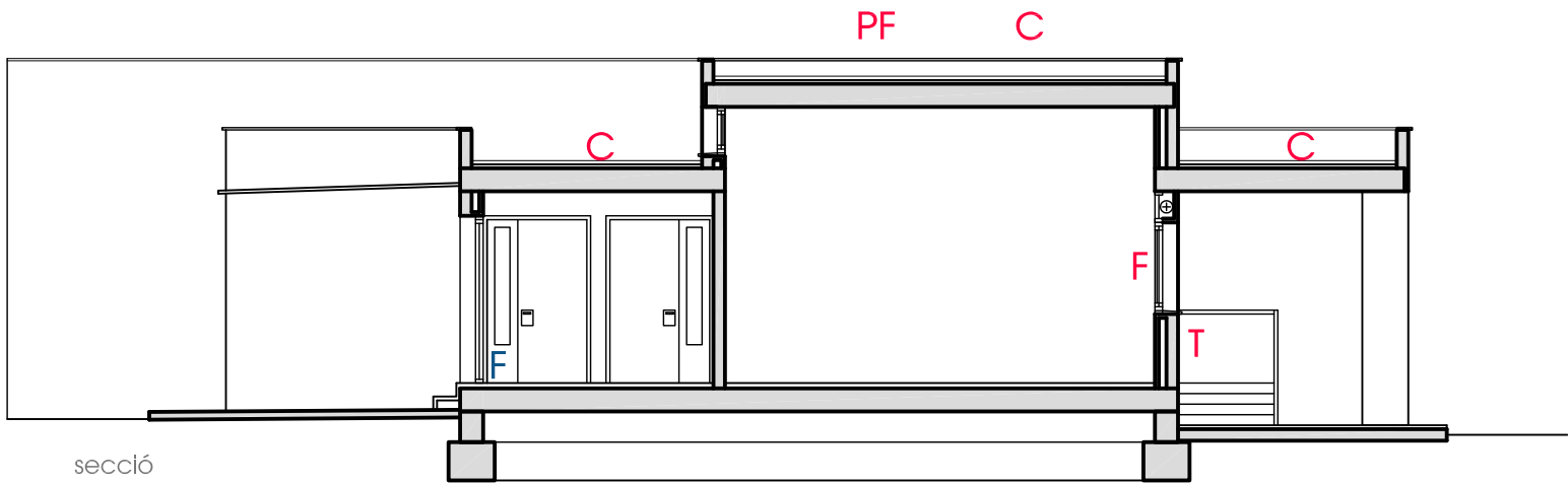
secció transversal
