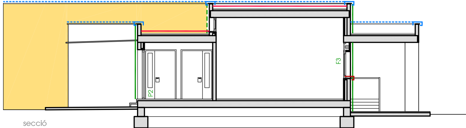
secció transversal
