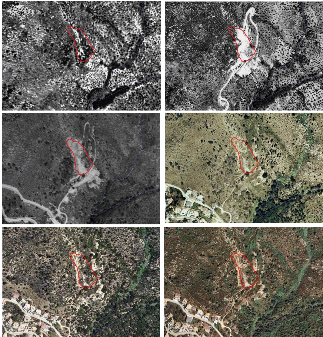
Figura 2 . Evolució de l'explotació minera sobre ortofotomapa del ICGC
